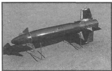
Ракета комплекса «Корнет-Э» и ее ТПК
