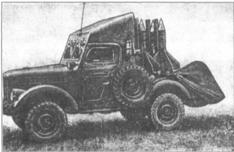
Боевая машина 2П26 комплекса «Шмель» в походном положении (тент опущен)
