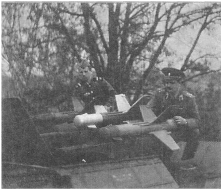
Установка ПТУР «Фаланга» на 9П32
