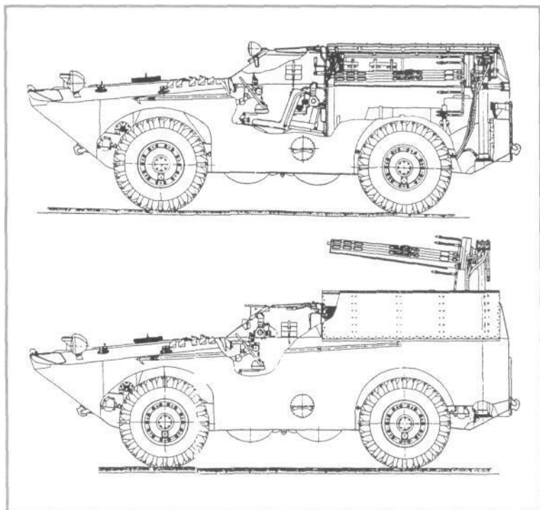
Боевая машина 2П27 комплекса «Шмель»
