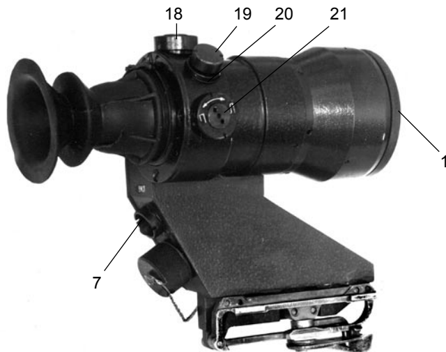
Рисунок 2 – Прицел (вид справа)
