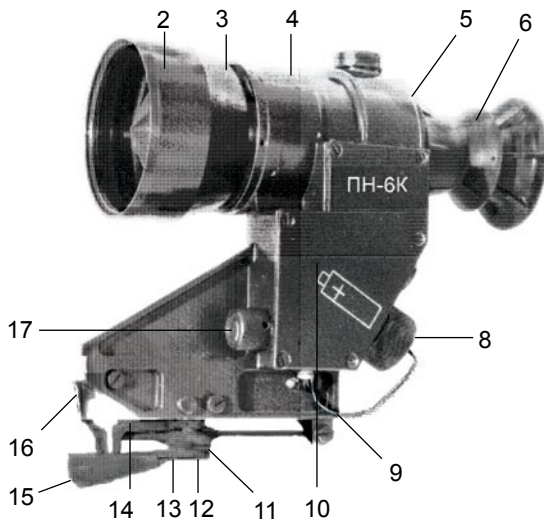
Рисунок 1 – Прицел (вид слева) без крышки со светофильтром
