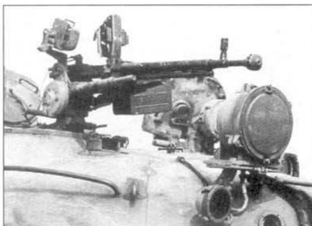
Крупный план зенитного пулемета ДШК-М, установленного на танке Т-62 (обр. 1972 г.). Хорошо видны НК прожекторы и амбразура спаренного пулемета.
