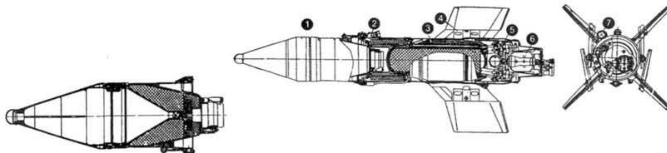
Компоновочная схема ракеты 9М14 комплекса «Малютка». Цифрами обозначены: 1 - боевая часть; 2 - двигательная установка; 3 - катушка; 4 - крыльевой отсек; 5 - рулевая машинка; 6 - гироскоп; 7 - трассер.
