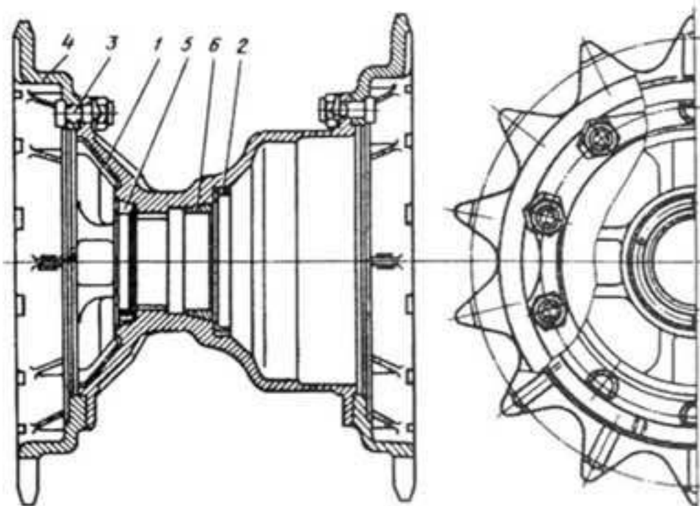
Вверху: Ведущее колесо для металлической гусеницы (14 зубьев). Цифрами обозначены: 1 - ступица; 2 - кольцо; 3 - болт; 4 - венец; 5 - наружный конус; 6 - внутренний конус.
