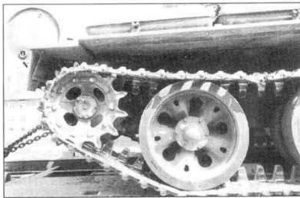
Кормовая часть танка Т-62. Видны задние опорные катки и ведущее колесо металлической гусеницы (имет 13 зубьев). Также хорошо видны наружный топливный бак и сзади дополнительные топливные бочки (укрепленные на специальных кронштейнах).
