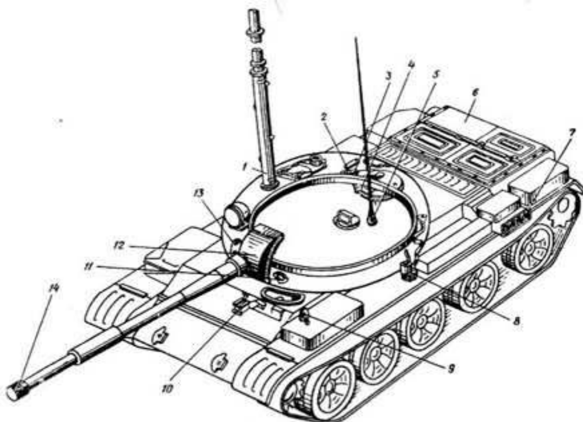
Комплект ОПВТ, установленный на танке Т-62.
