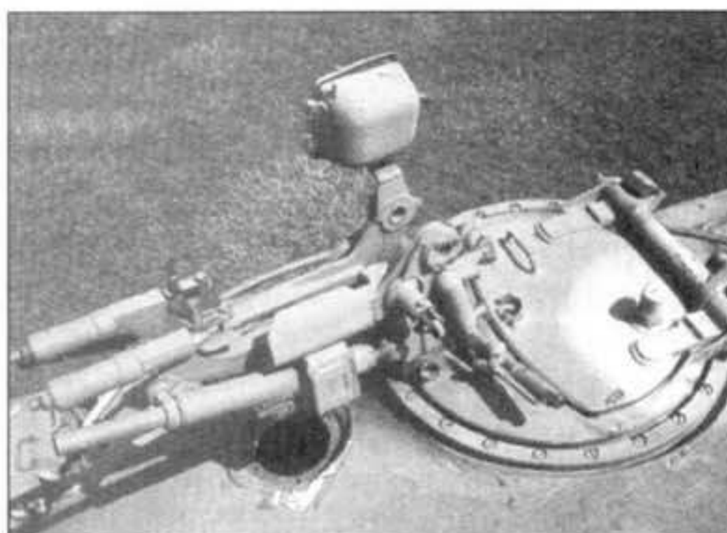
Зенитная турель на танке Т-62 (обр. 1972 г.). Хорошо видны крышка люка заряжающего, турель, лафет для пулемета. В коробке (в верхней части лафета) находится зенитный прицел К-10Т.
