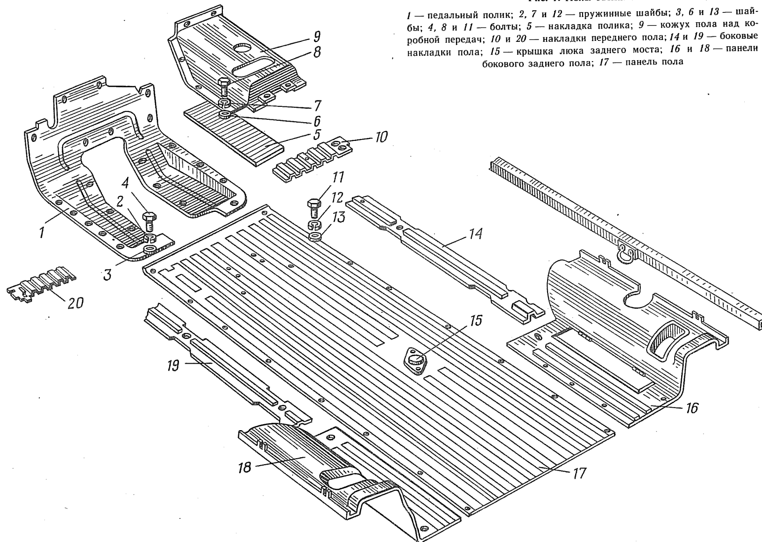
Рис. 1. Полы съемные:
