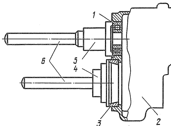
Рис. 173. Запрессовка наружных подшипников колесного редуктора:
