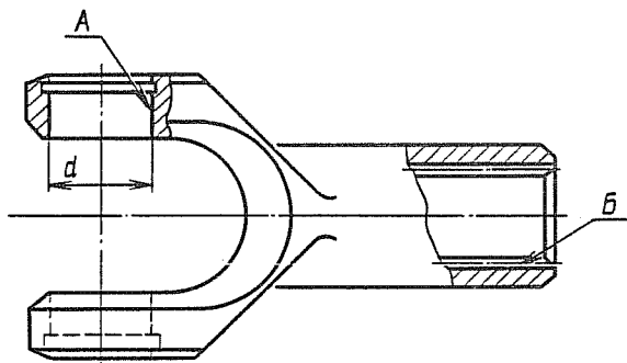
Рис. 194. Вилка верхняя карданного вала
