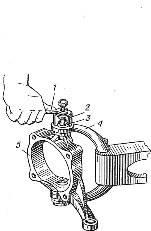
Рис. 74. Выпрессовка шкворня поворотного кулака:
