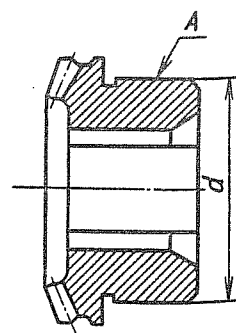
Рис. 145. Шестерня полуоси
