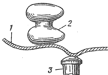
Рис. 222. Быкотка вмятин: 1 — деталь; 2 — поддержка; 3 — выкоточный молоток
