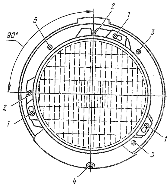
Рис. 95. Фара:
