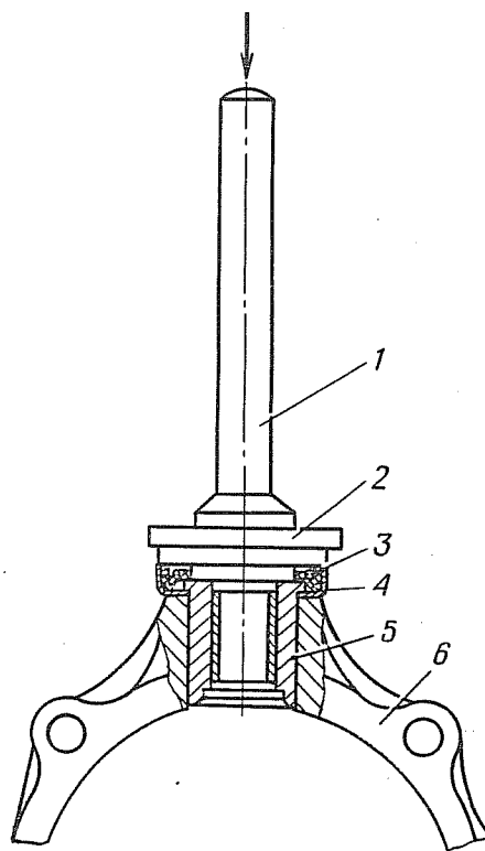
Рис. 77. Запрессовка сальника шкворня:
