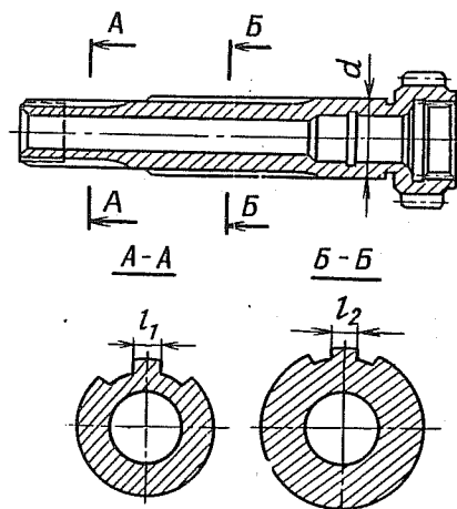
Рис. 140. Промежуточный вал коробки передач
