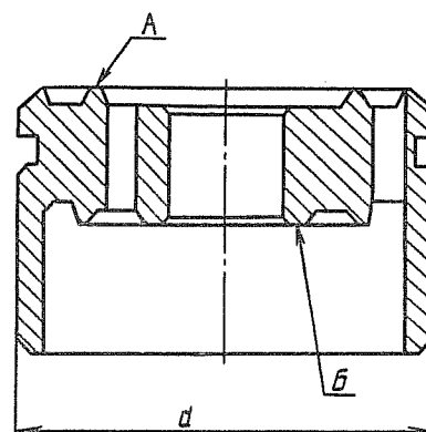
Рис. 183. Поршень амортизатора
