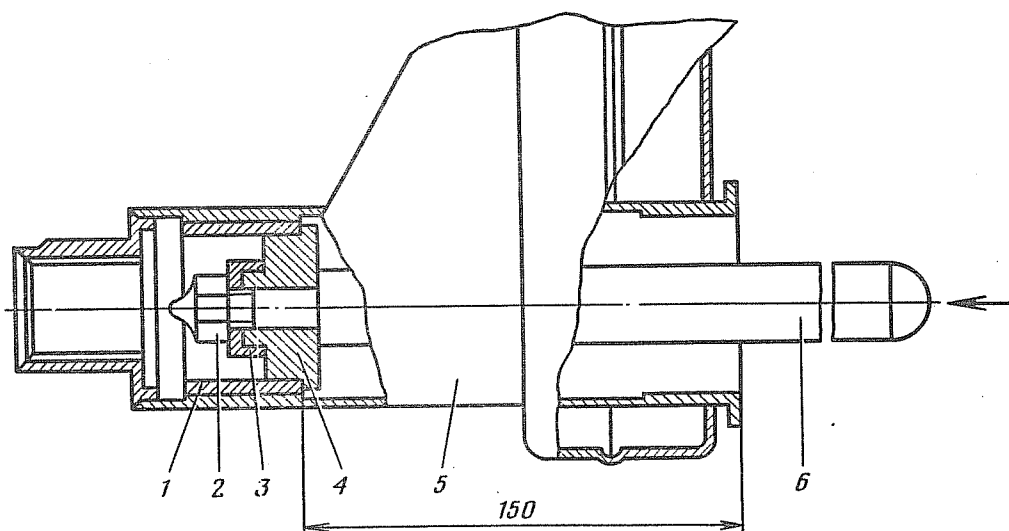
Рис. 68. Запрессовка наружной втулки рычага подвески:
