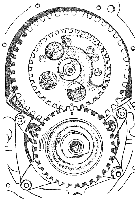
Рис. 32. Совмещение меток шестерен привода балансирующего вала
