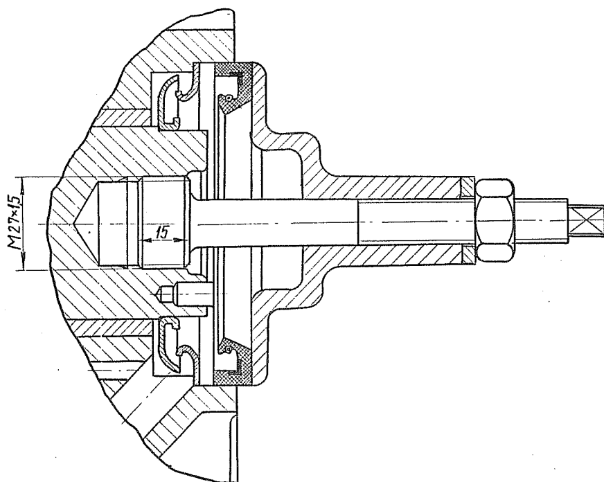
Рис. 21. Оправка для запрессовки сальника коленчатого вала со стороны маховика
