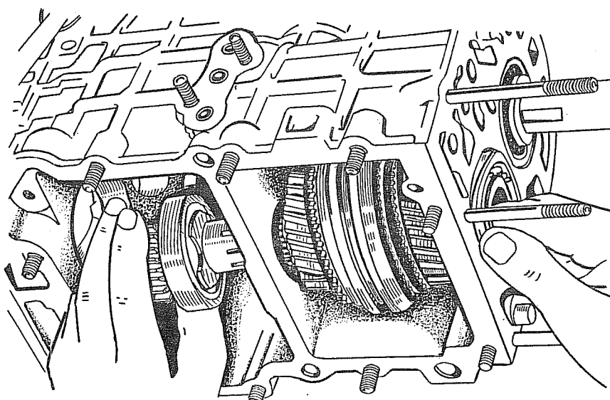
Рис. 152. Установка промежуточного вала
