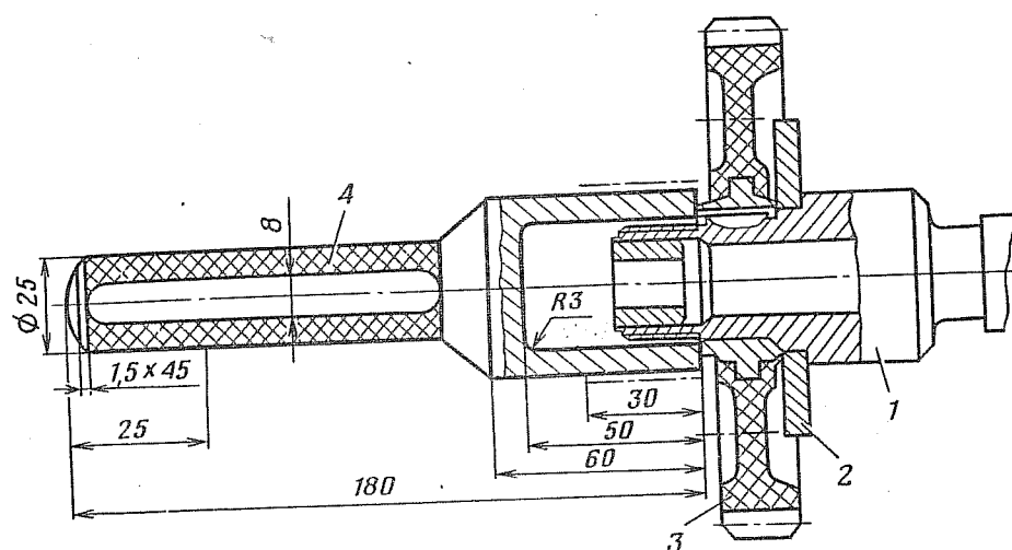
Рис. 31. Оправка для напрессовки шестерни распределительного вала:
