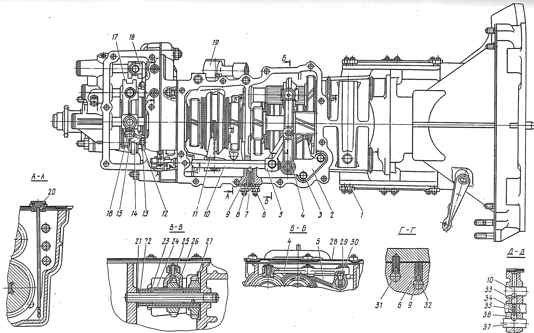
Рис. 131. Коробка передач (вид сверху):
