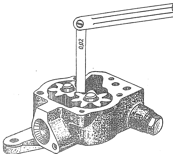
Рис. 106. Проверка бокового зазора между зубьями шестерен масляного насоса
