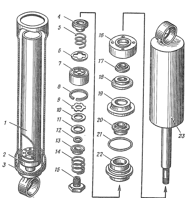
Рис. 180. Амортизатор в сборе (11.2915006):
