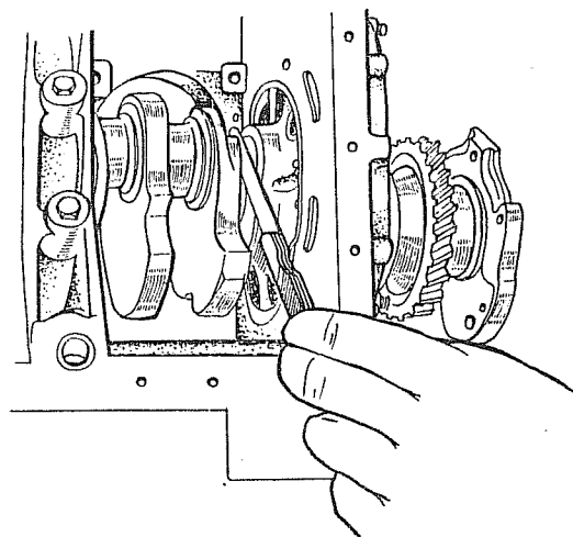
Рис. 27. Проверка осевого перемещения коленчатого вала
