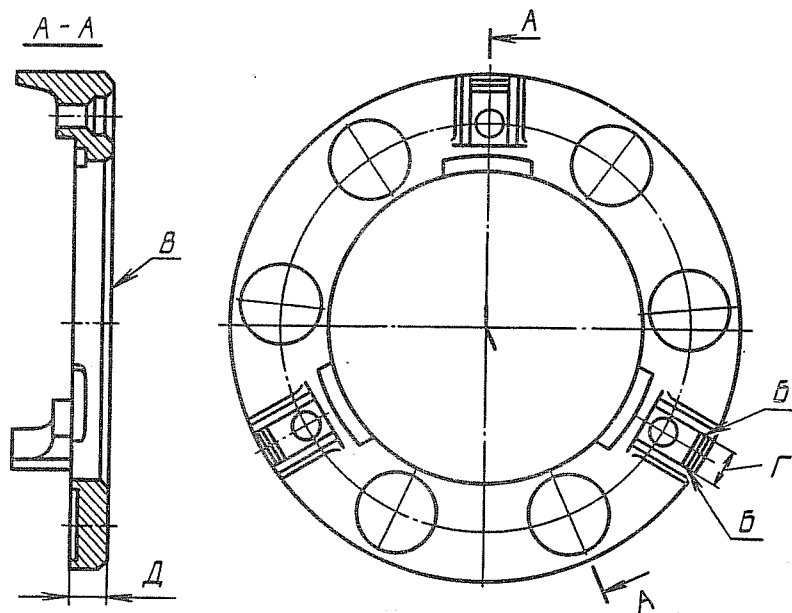
Рис. 124. Нажимной диск
