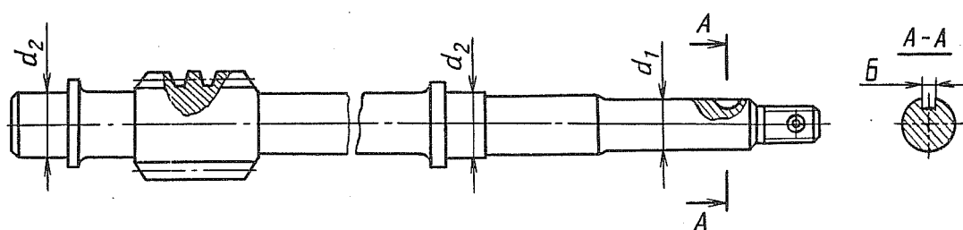
Рис. 211. Червяк редуктора лебедки
