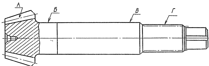
Рис. 175. Ведущая шестерня главной передачи
