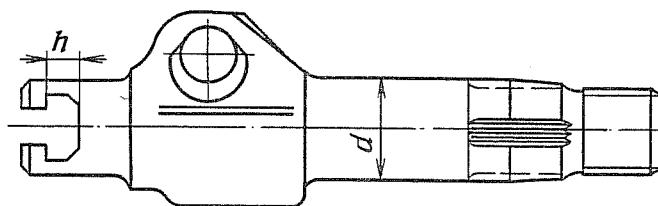
Рис. 189. Вал сошки рулевого управления
