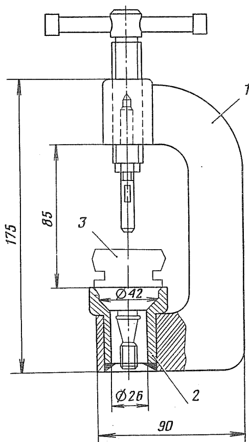
Рис. 185. Приспособление для разборки и сборки шаровых шарниров:
