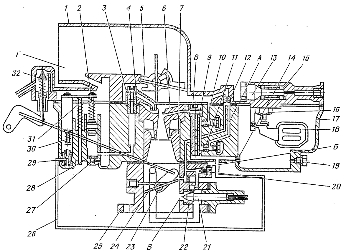
Рис. 118. Схема карбюратора К-133А:
