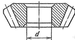
Рис. 144. Сателлит дифференциала
