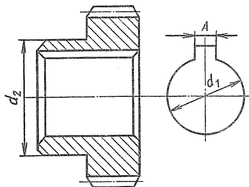
Рис. 214. Ступица ведомого диска привода лебедки
