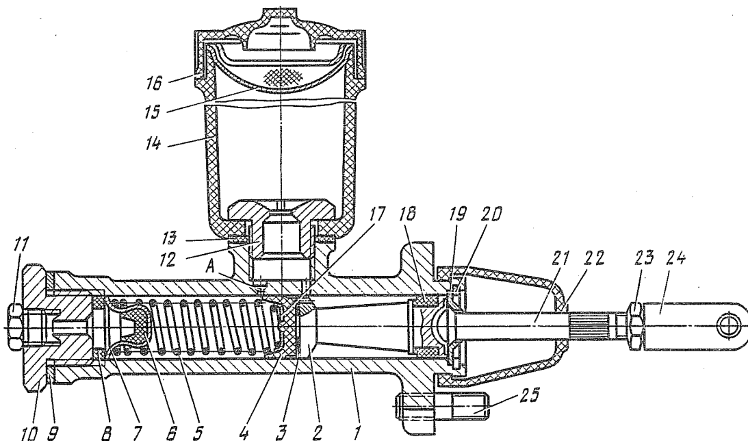
Рис. 199. Главный цилиндр тормоза:
