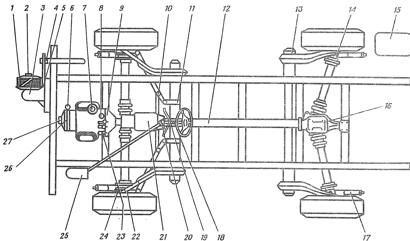
Рис. 220. Схема смазывания
