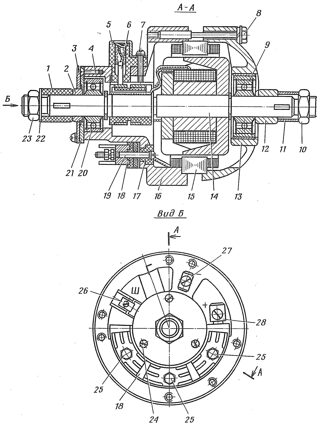
Рис. 201. Генератор:
