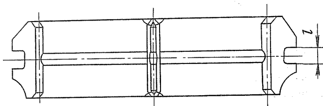
Рис. 146. Муфта включения синхронизатора 3-й и 4-й передач
