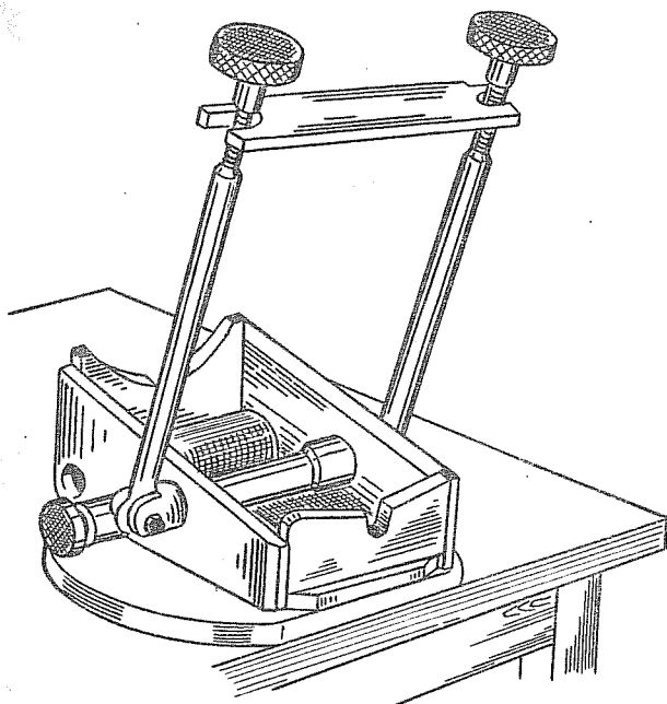
Рис. 57. Приспособление для разборки и сборки коробки передач
