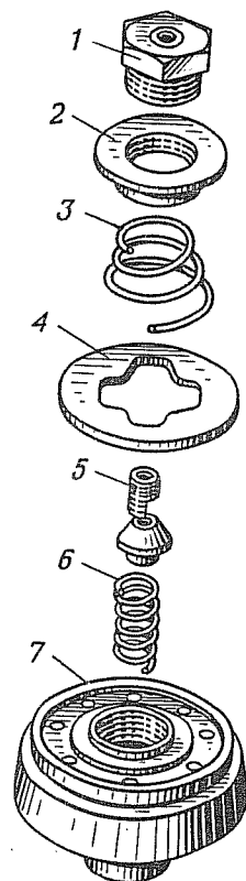
Рис. 181. Клапан сжатия амортизатора:
