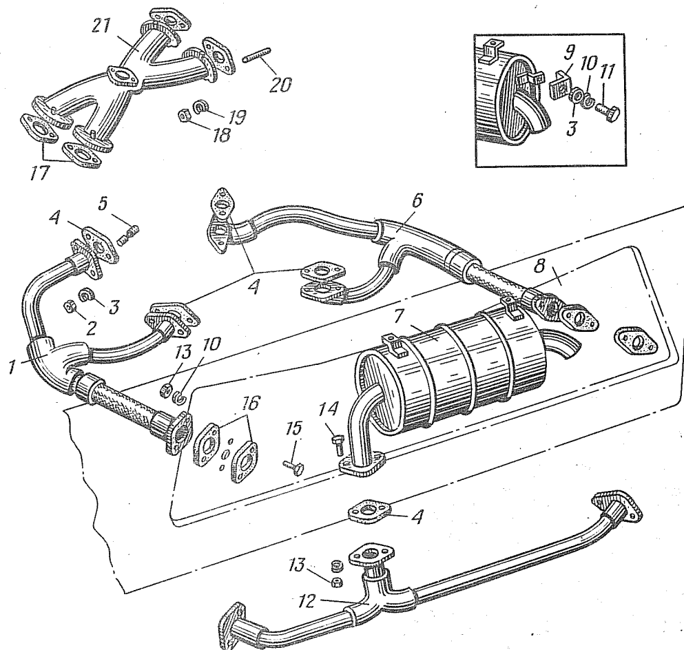
Рис. 38. Система впуска и выпуска газов:
