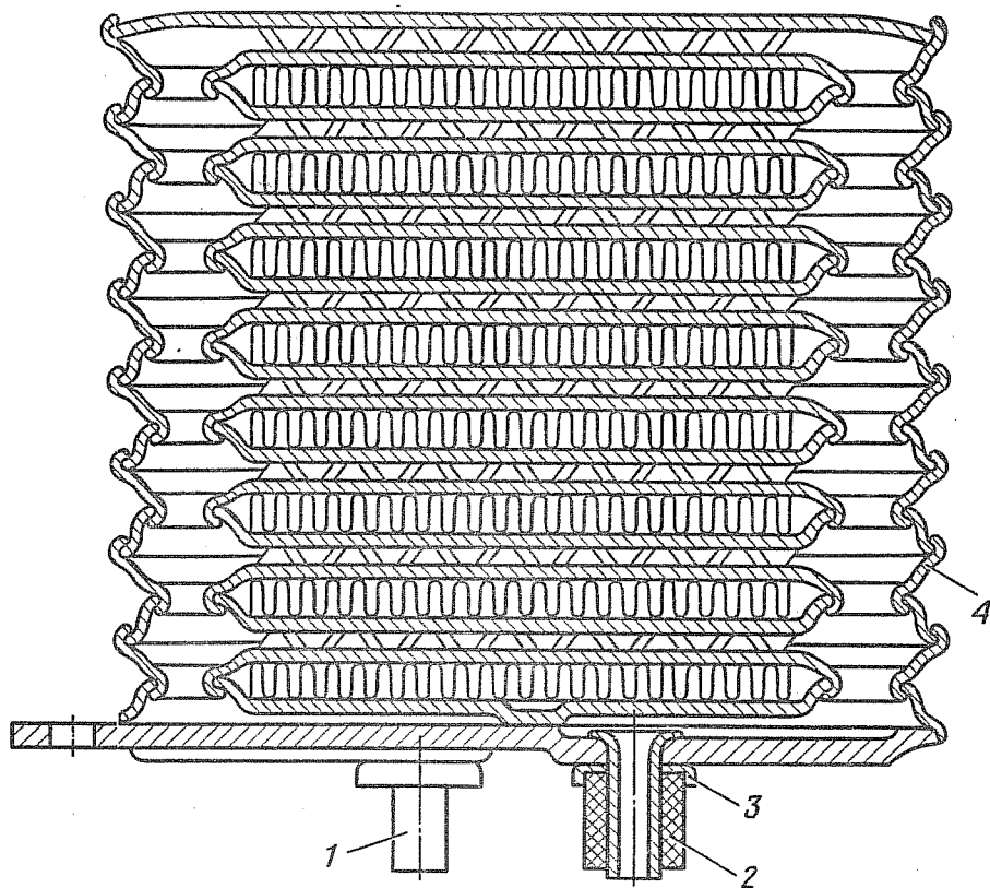
Рис. 40. Масляный радиатор:
