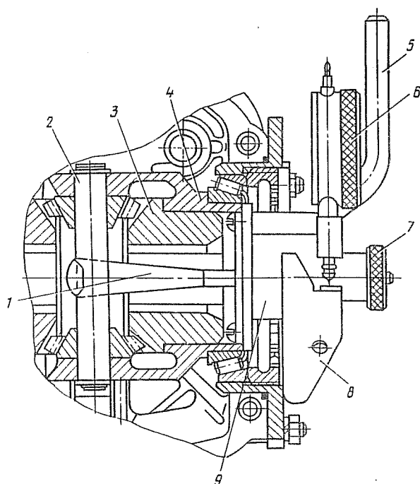
Рис. 153. Контроль бокового зазора в зацеплении шестерен главной передачи в редукторе заднего моста и коробке передач:
