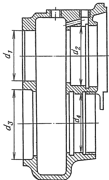
Рис. 169. Картер колесного редуктора
