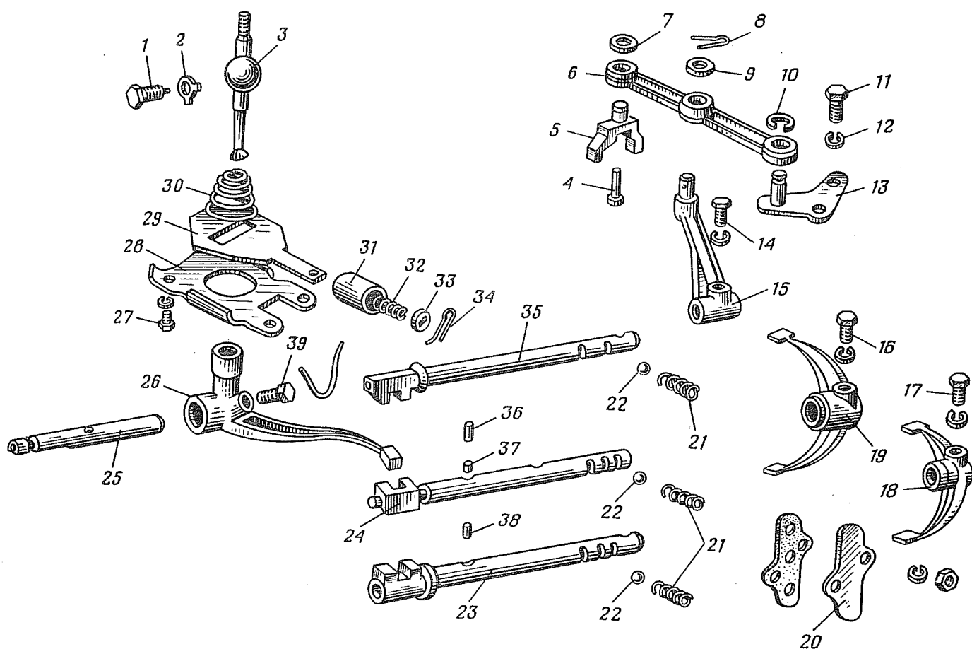
Рис. 134. Детали механизма переключения передач:
