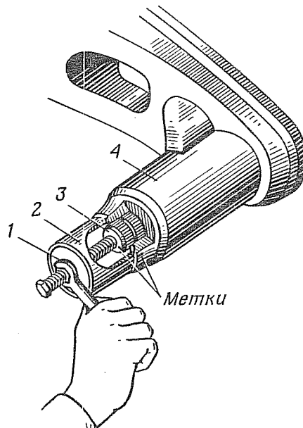
Рис. 69. Выпрессовка торсиона:
