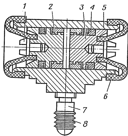
Рис. 197. Цилиндр колесный тормоза:
