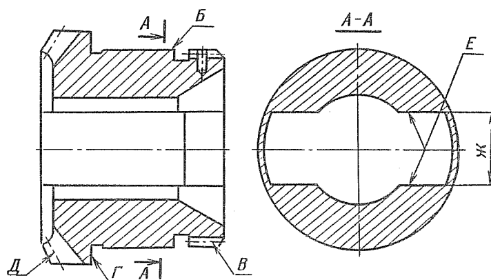
Рис. 177. Шестерня полуоси заднего моста левая
