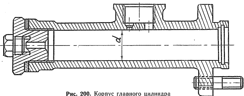
Рис. 200. Корпус главного цилиндра
