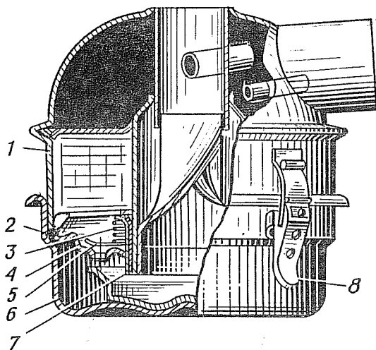
Рис. 121. Воздушный фильтр:
