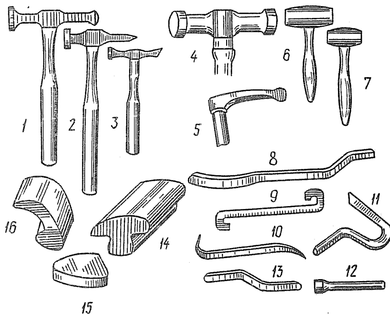
Рис. 223. Набор инструмента для устранения вмятин: 1, 2, 3, 4 и 5 — молотки; 6 и 7 — киянки; 8, 9, 10, 11, 12 и 13 — оправки; 14, 15 и 16 — поддержки
