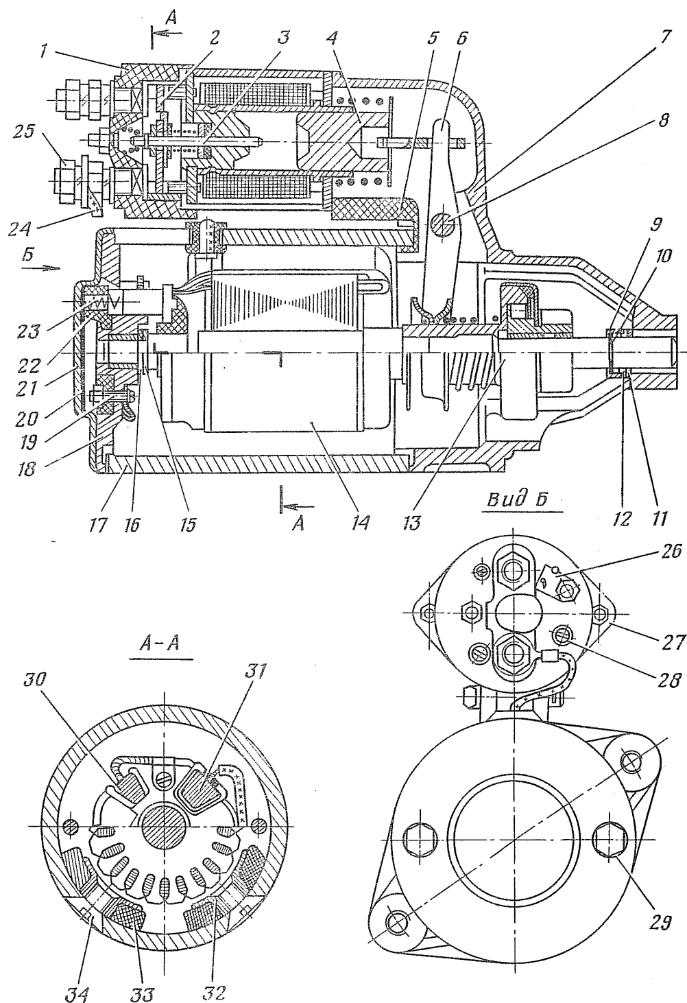
Рис. 206. Стартер:
