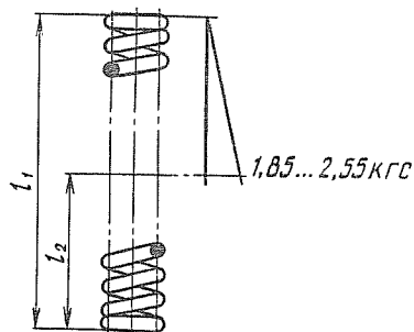
Рис. 104. Пружина редукционного клапана
