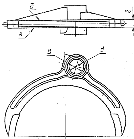
Рис. 147. Вилка включения 3-й и 4-й передач
