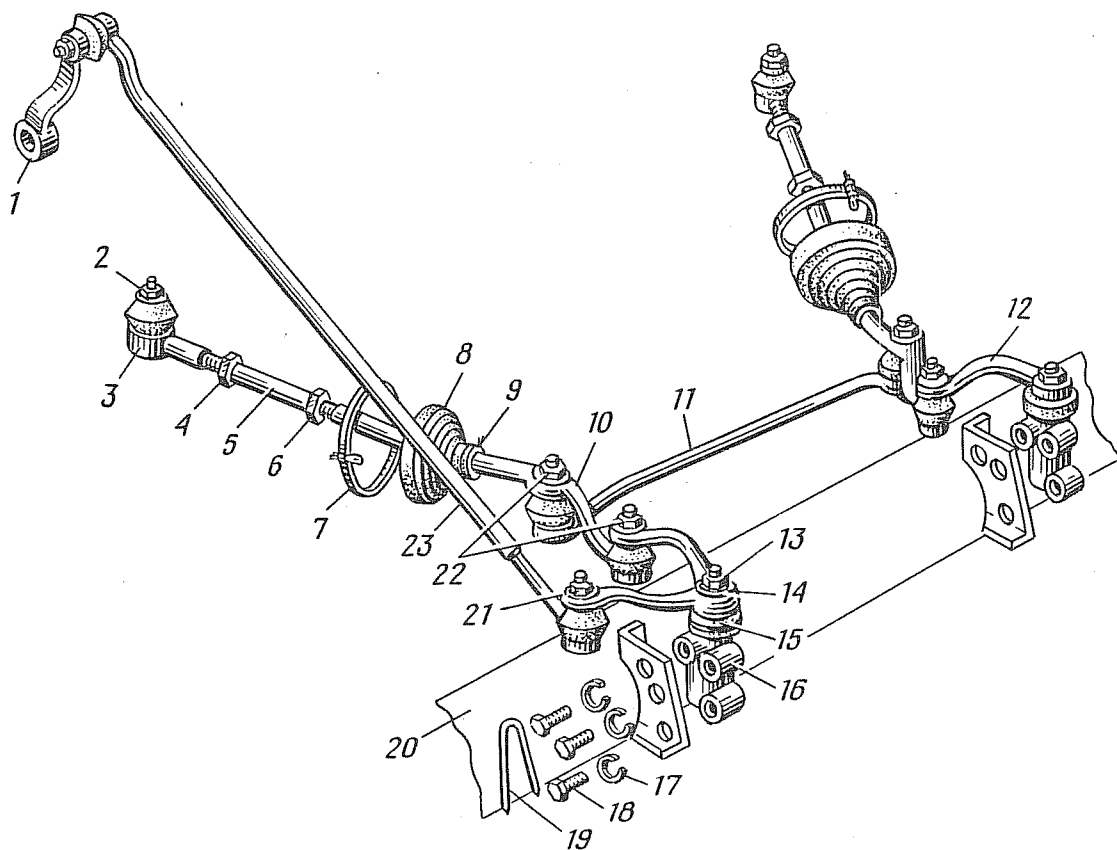
Рис. 78. Рулевой привод:
