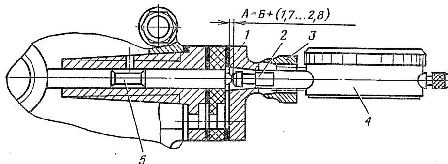
Рис. 47. Приспособление для замера выступающей штанги привода топливного насоса:
