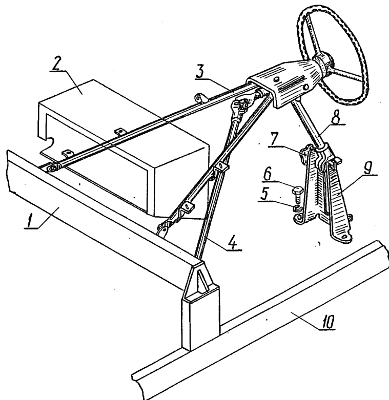
Рис. 2. Рулевое управление:
