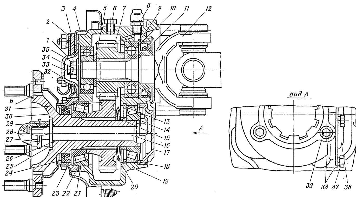
Рис. 166. Колесный редуктор:
