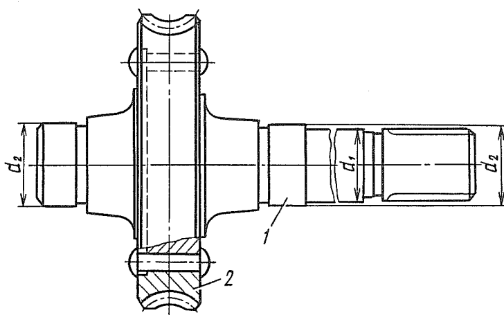
Рис. 212. Вал лебедки в сборе с червячным колесом: 1 — вал; 2 — червячное колесо
