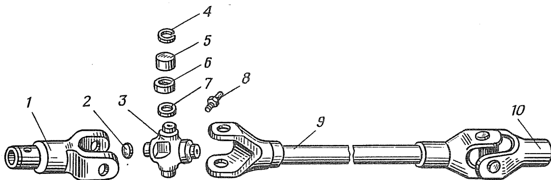
Рис. 192. Детали карданного вала рулевого управления:
