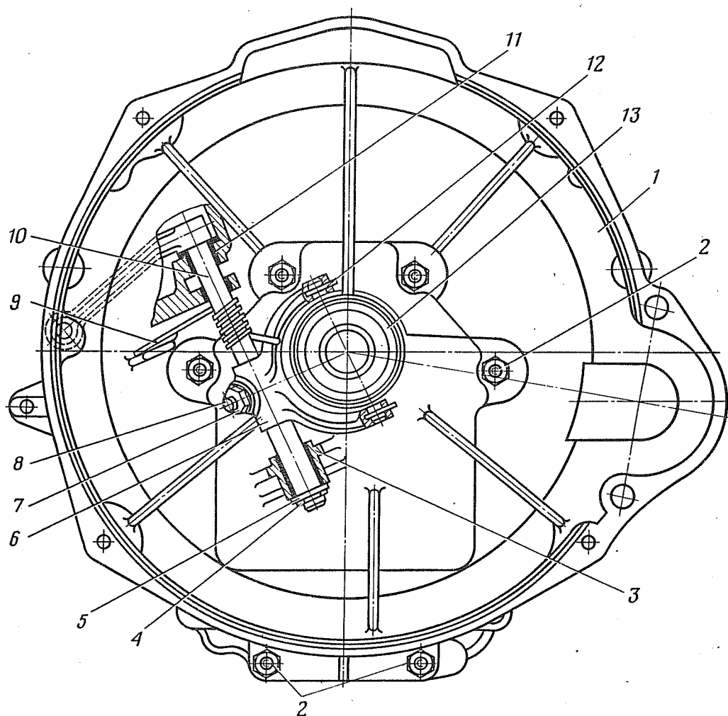
Рис. 52. Механизм выключения сцепления:
