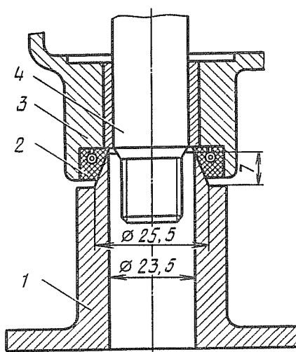
Рис. 188. Отжатие кромки сальника вала сошки при разборке и сборке рулевого механизма:
