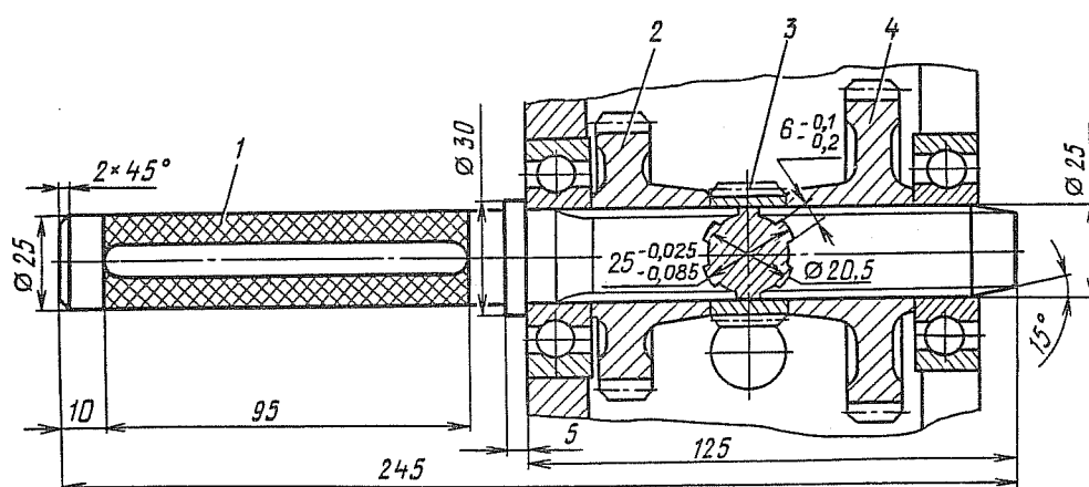
Рис. 151. Оправка для удержания шестерен:
