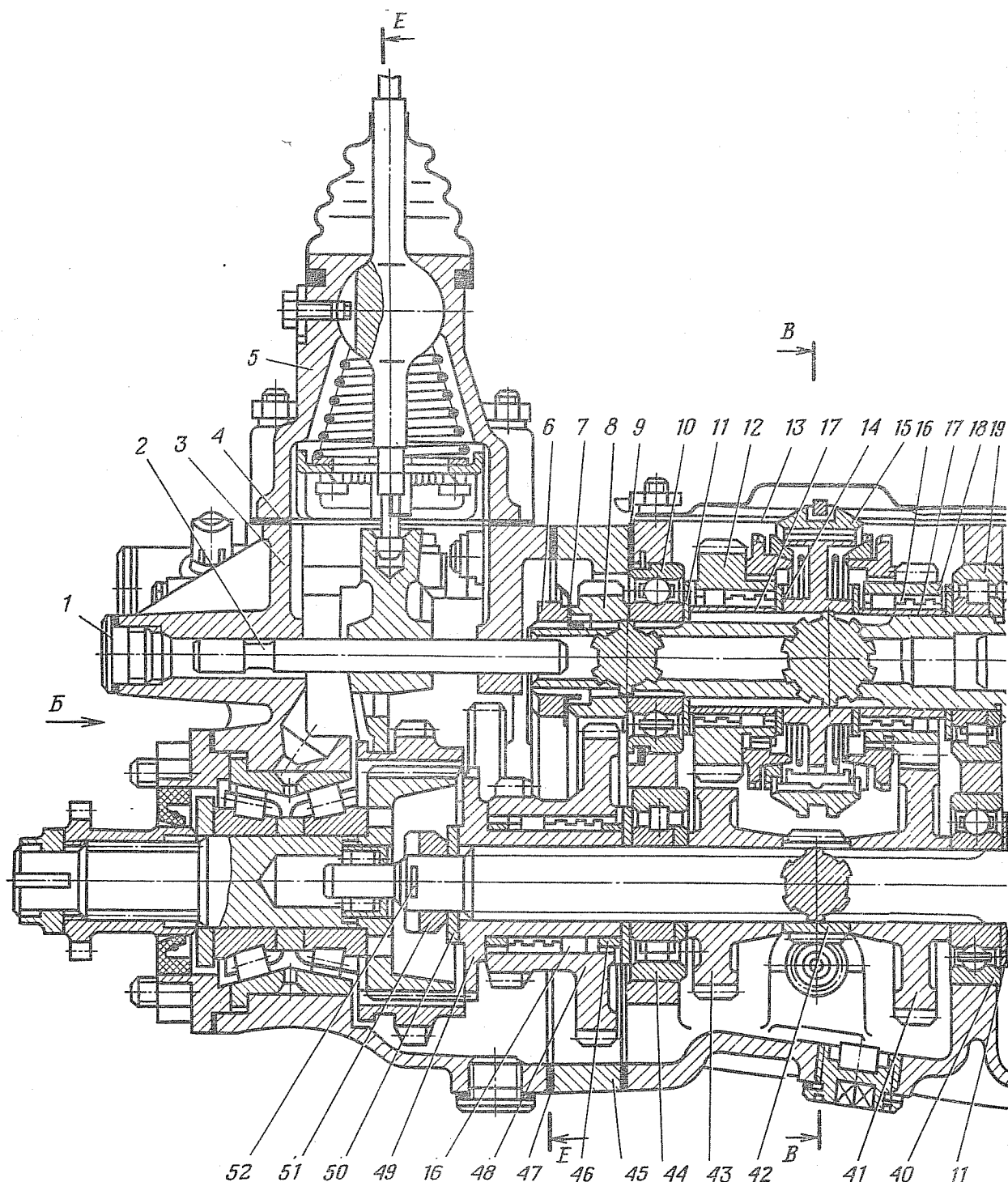
Рис. 132. Коробка передач (вид сбоку;
