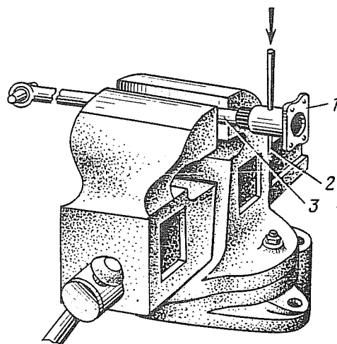
Рис. 161. Выпрессовка стопорного штифта фланца полуоси:
