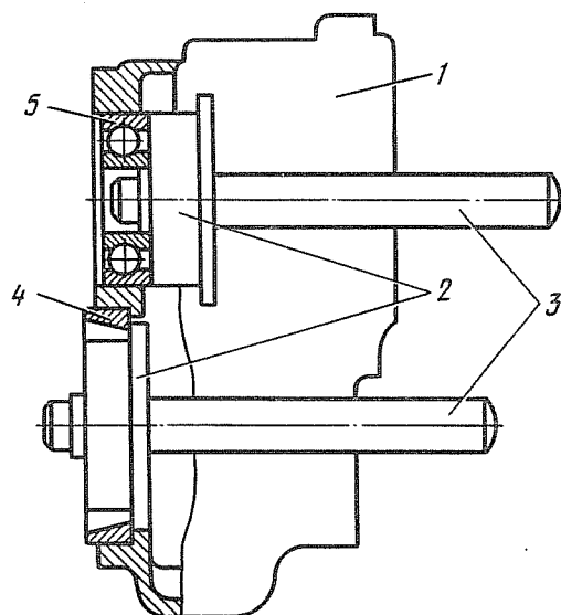
Рис. 168. Выпрессовка наружных подшипников колесного редуктора:
