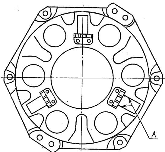
Рис. 128. Кожух сцепления
