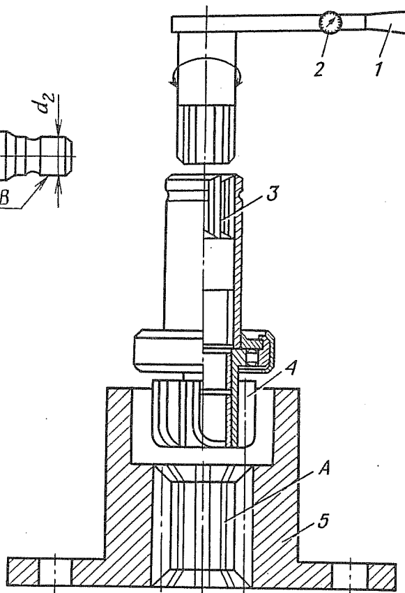
Рис. 208. Приспособление для проверки муфты свободного хода:
