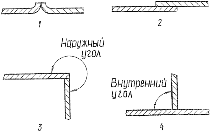
Рис. 227. Виды сварных соединений: 1 — встык с отбортовкой; 2 — внахлестку; 3 — угловое; 4 — тавровое
