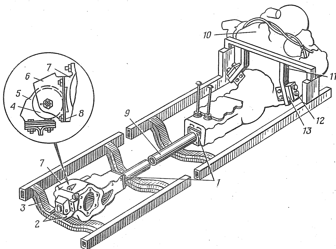
Рис. 5. Подвеска силового агрегата и редуктора заднего моста:
