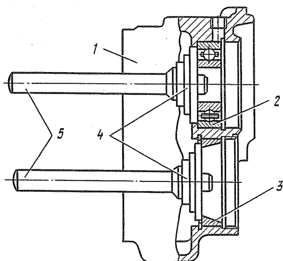
Рис. 167. Выпрессовка внутренних подшипников колесного редуктора:
