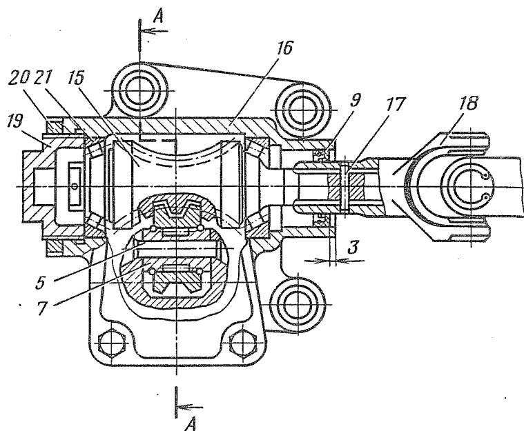
Рис. 187. Рулевой механизм в сборе:
