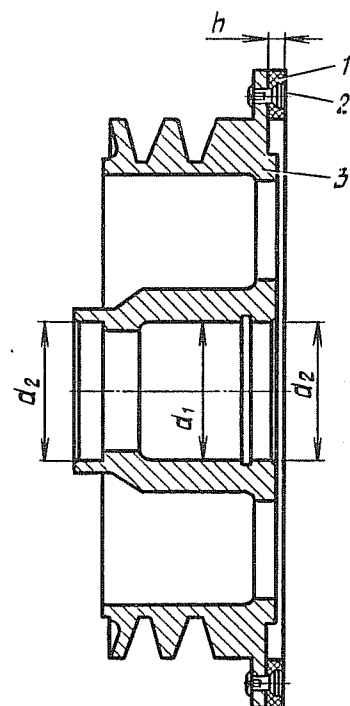
Рис. 213. Шкив привода лебедки в сборе: 1 — фрикционная накладка; 2 — заклепка; 3 — шкив
