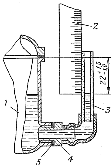
Рис. 120. Проверка уровня топлива в поплавковой камере карбюратора:
