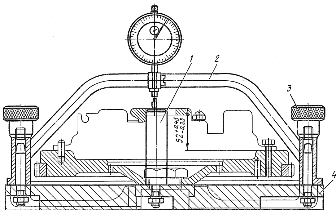
Рис. 51. Приспособление для регулировки положения пяты сцепления:
