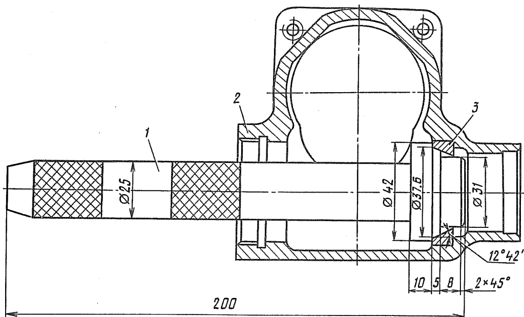
Рис. 191. Запрессовка наружного кольца подшипника червяка рулевого управления:
