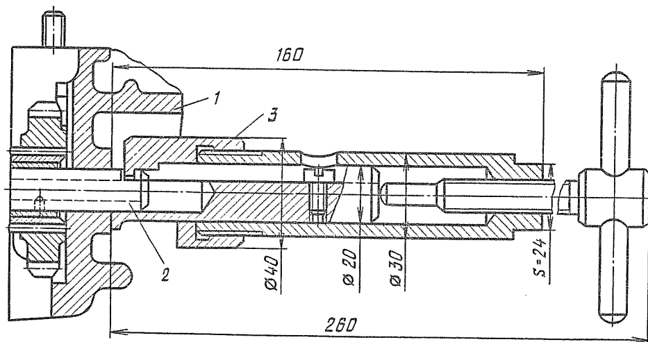
Рис. 135. Выпрессовка оси шлицевого вала:
