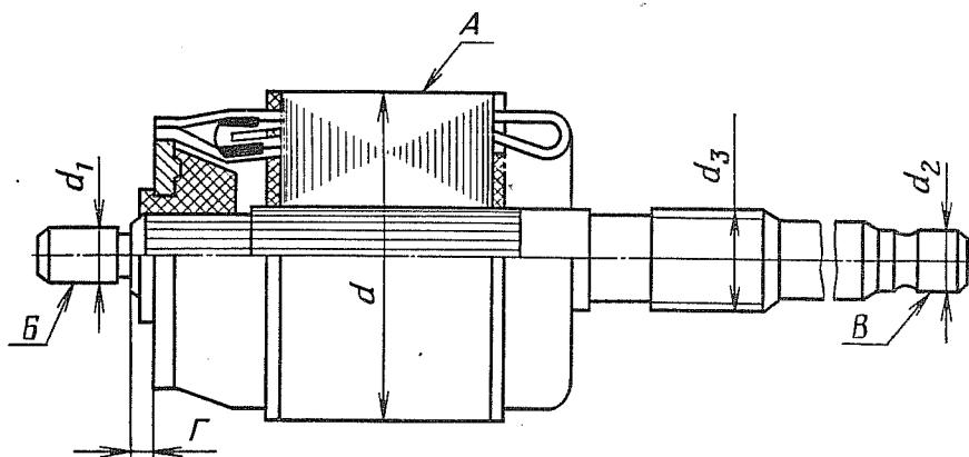
Рис. 207. Якорь стартера
