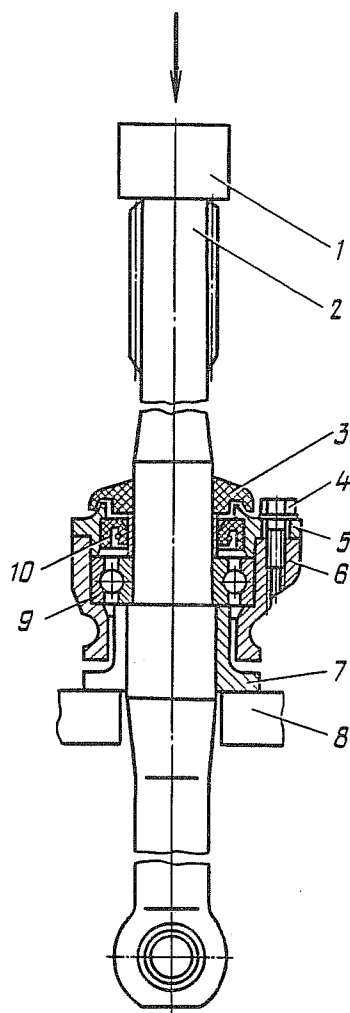
Рис. 162. Спрессовка с полуоси подшипникового узла:
