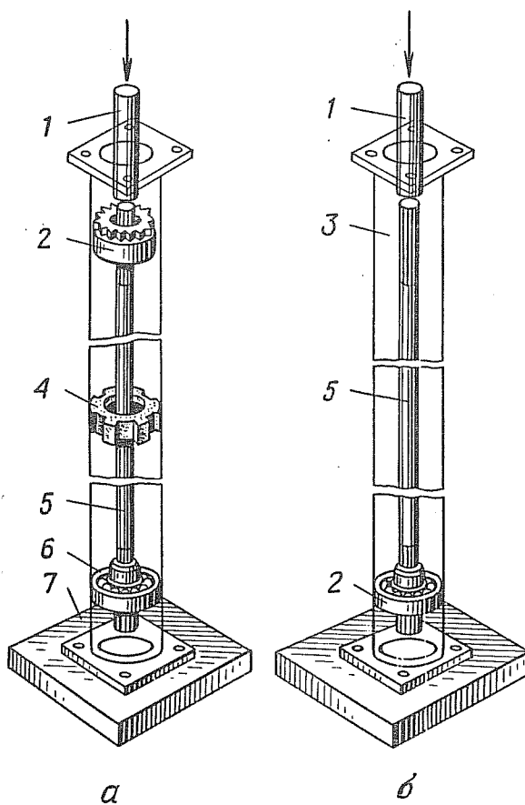
Рис. 155. Разборка приводного вала:
