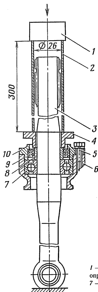
Рис. 164. Напрессовка на полуось подшипникового узла:
