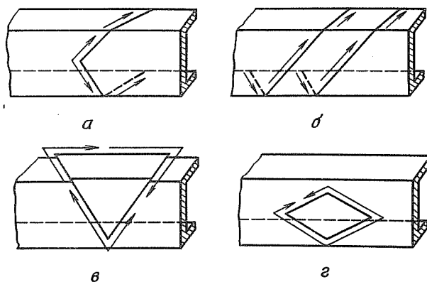
Рис. 228. Схема приварки надставок, вставок, накладок
