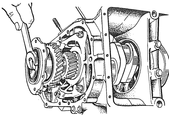
Рис. 28. Проверка проворачивания коленчатого вала
