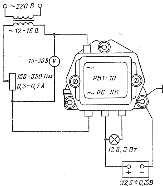
Рис. 89. Схема соединений для проверки реле блокировки
