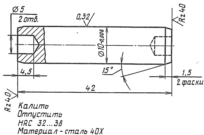
Рис. 190. Ось ролика вала сошки рулевого управления
