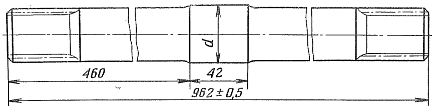
Рис. 159. Приводной вал
