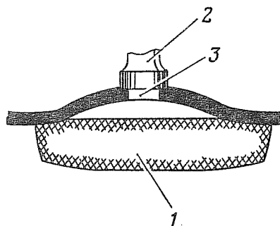
Рис. 225. Нагрев и осаждение выступов: 1 — поддержка; 2 — молоток; 3 — де- таль (место нагрева)
