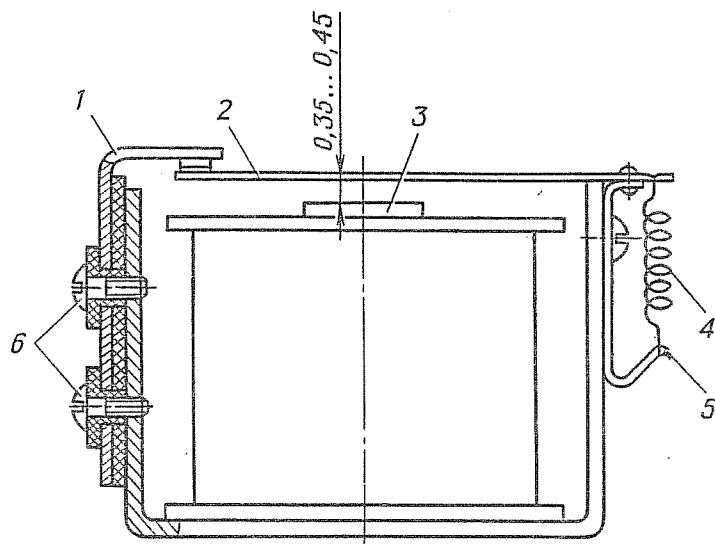
Рис. 90. Реле блокировки:
