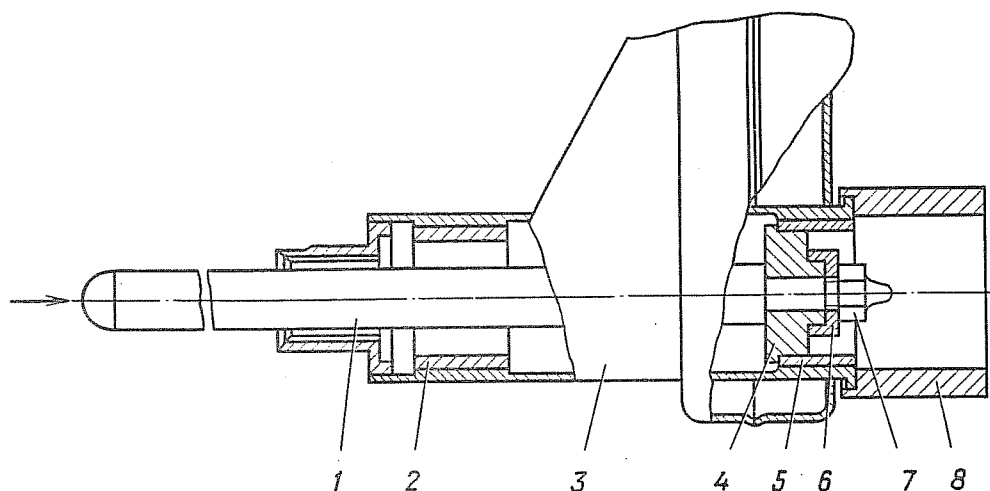
Рис. 67. Выпрессовка внутренней втулки рычага подвески:
