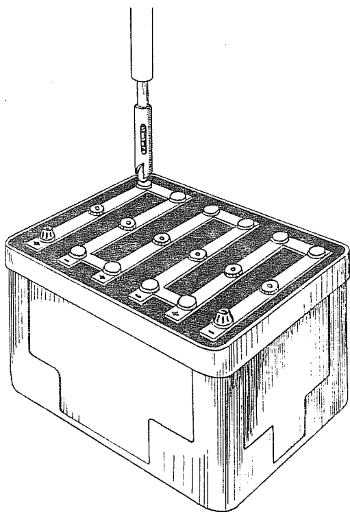
Рис. 202. Высверливание межэлементных соединений
