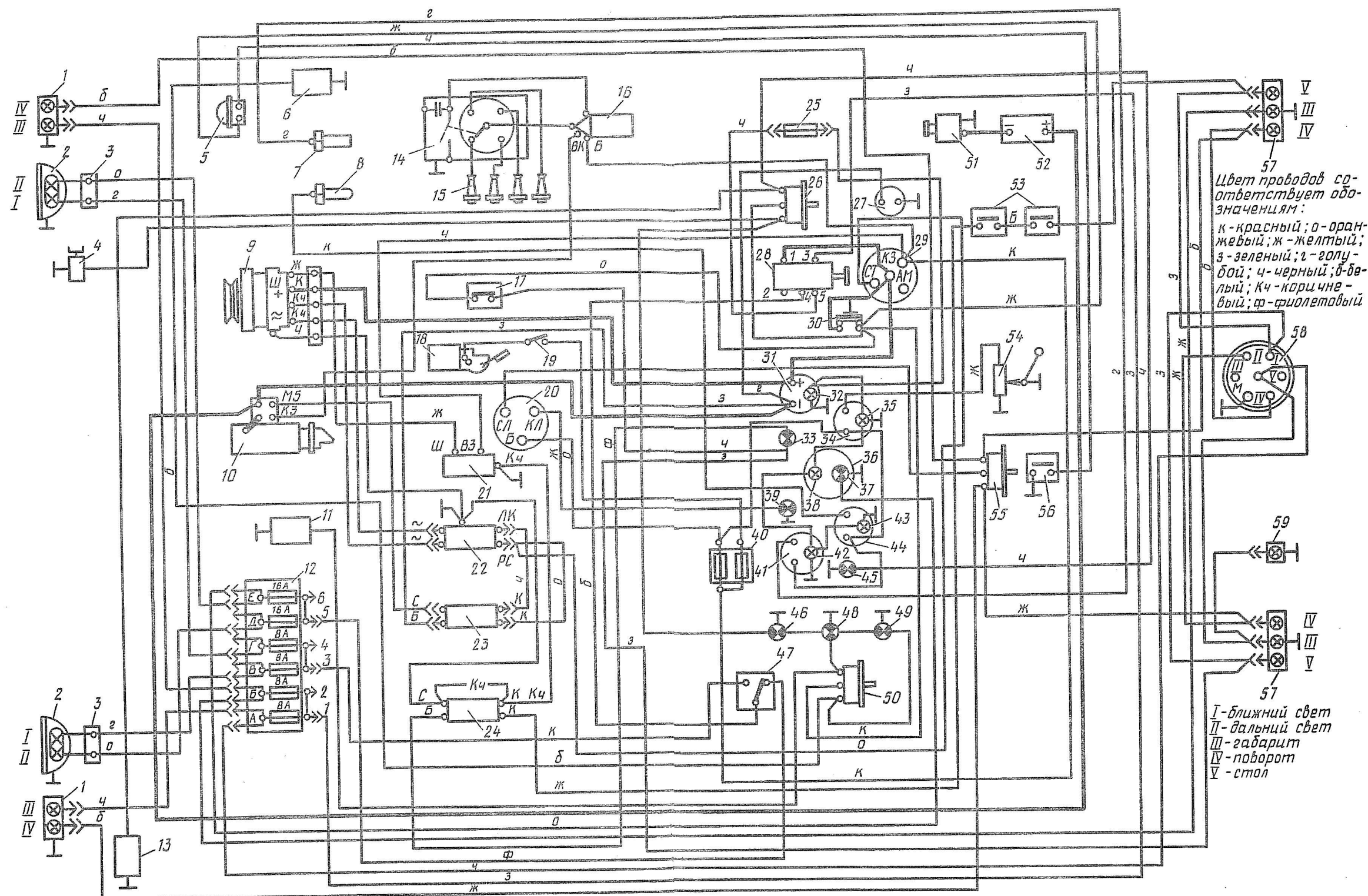
Рис. 221. Принципиальная схема
