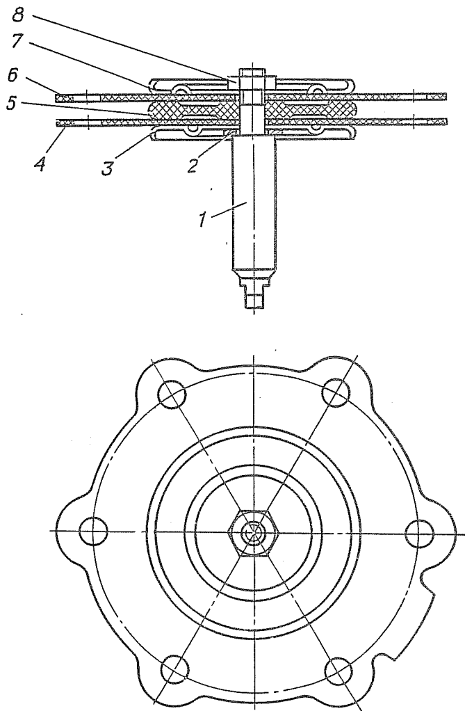
Рис. 114. Диафрагма топливного насоса в сборе:
