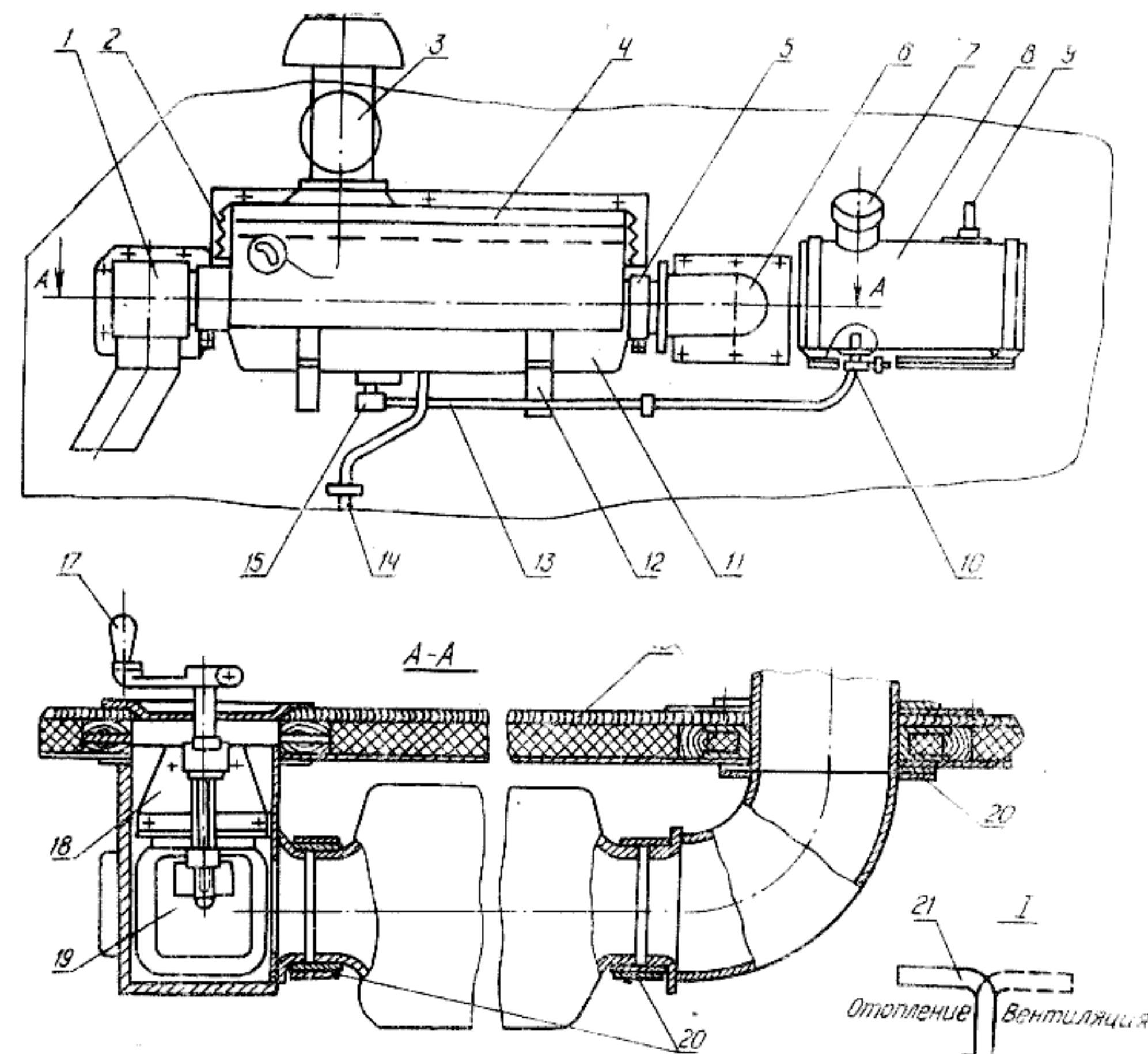
Рис. 7. Система отопления:
