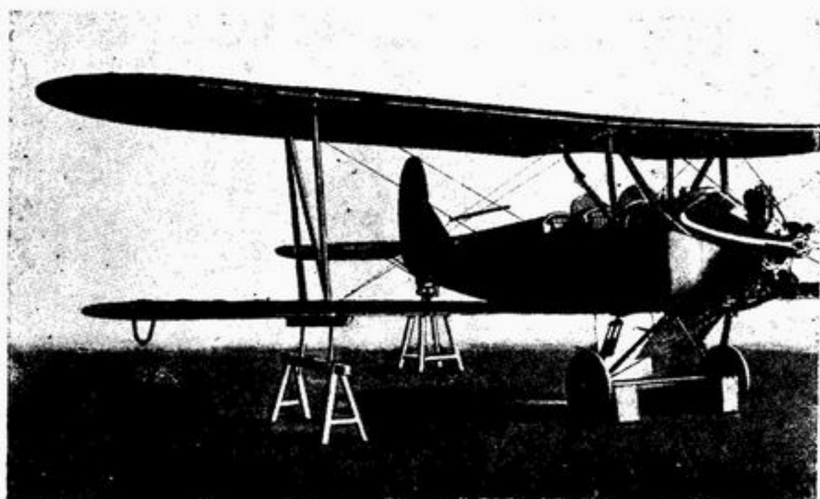
Рис. 227. Сборка коробки крыльев
