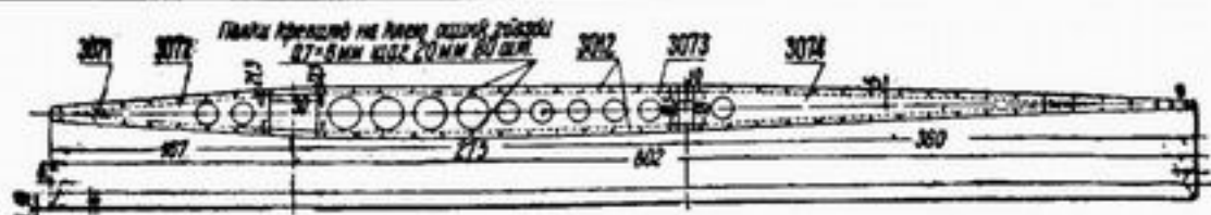
Рис. 126. Нервюра № 1
