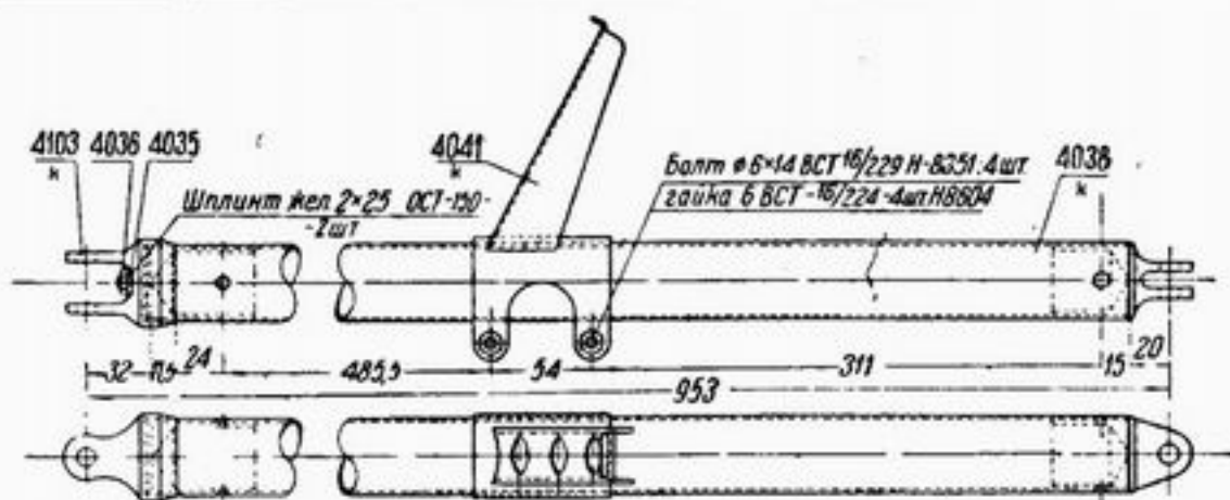
Рис. 159. Передняя нога
