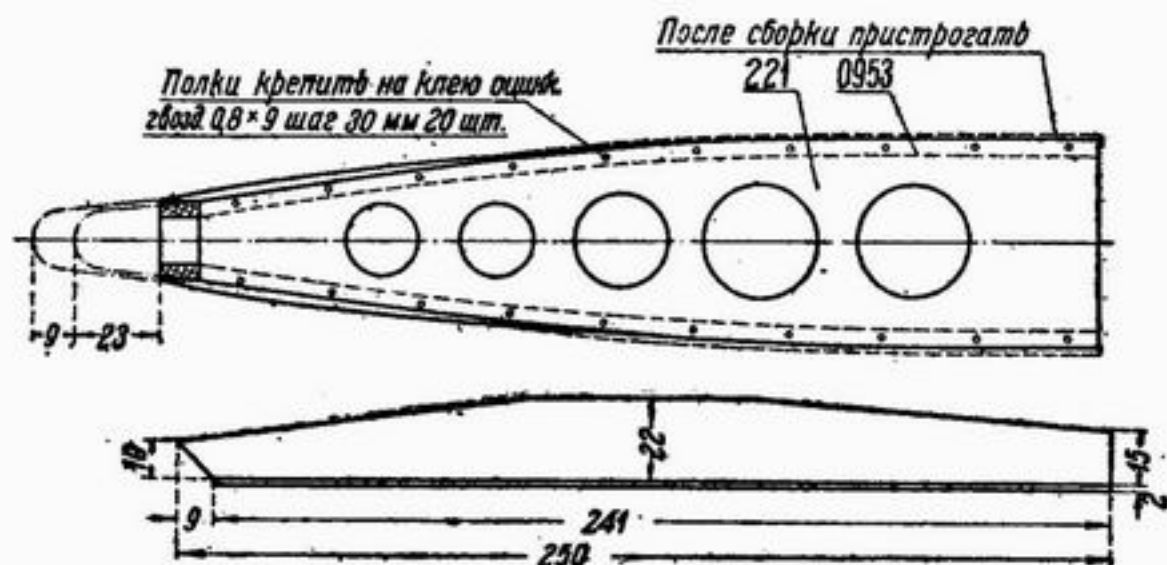
Рис. 46. Нервюра № 1
