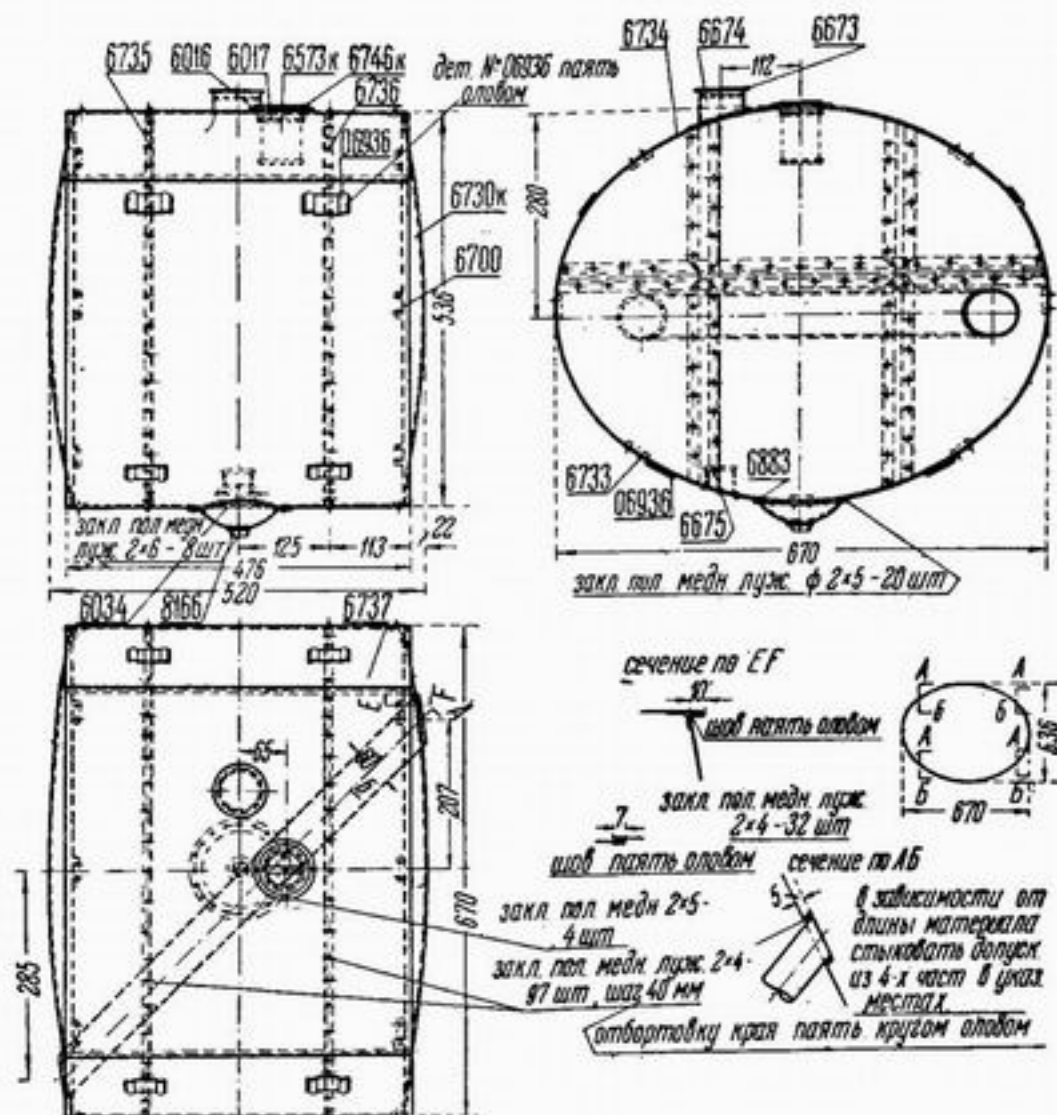
Рис. 186. Бензиновый бак
