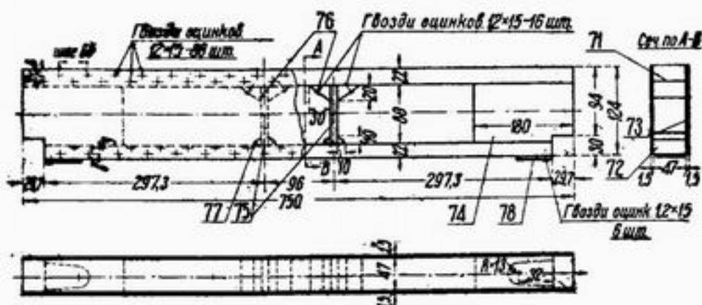
Рис. 19. Тело заднего поперечного лонжерона
