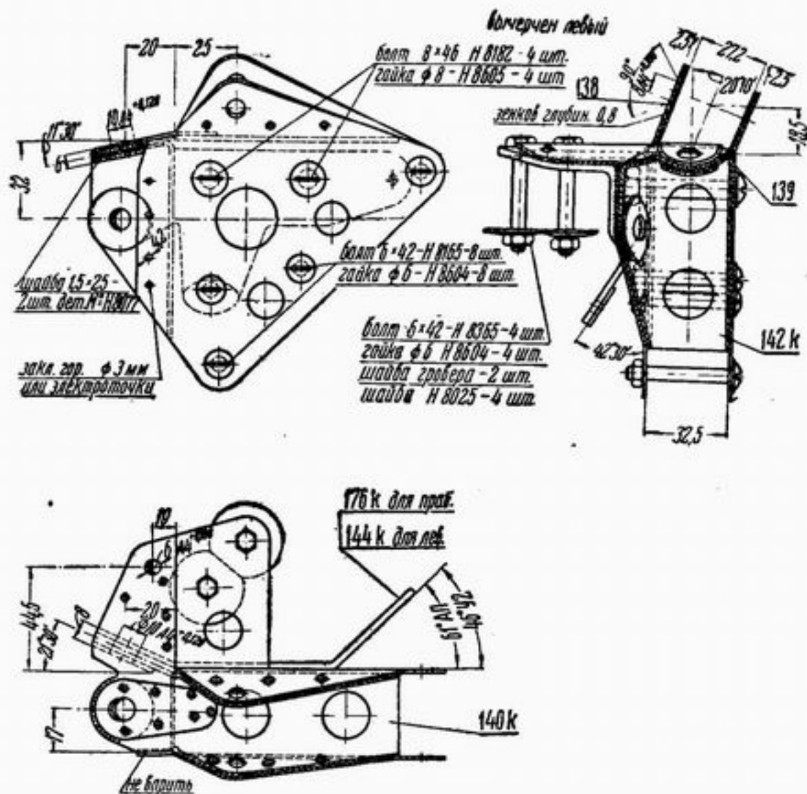
Рис. 22. Передний узел крепления кабана и мотогамы
