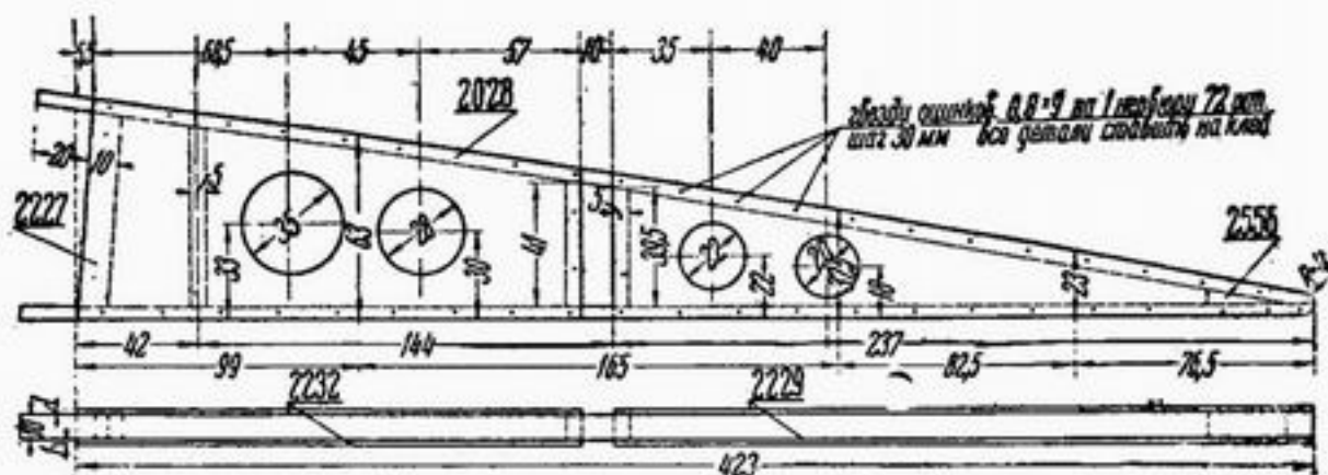
Рис. 99. Коробчатая нервюра
