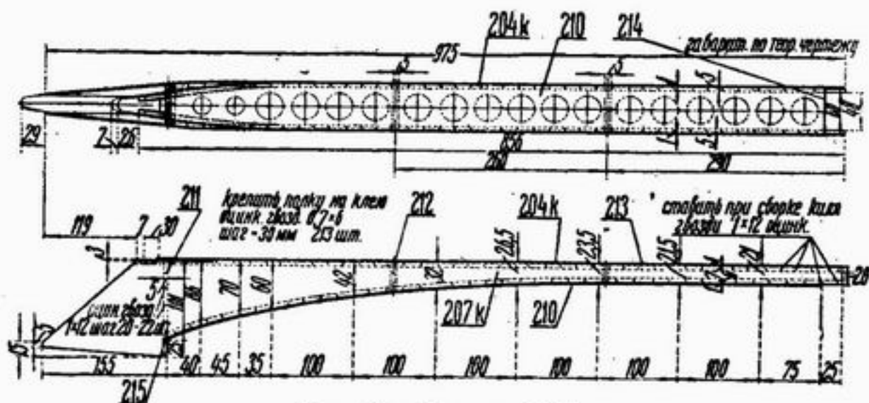
Рис. 48. Нервюра № 3
