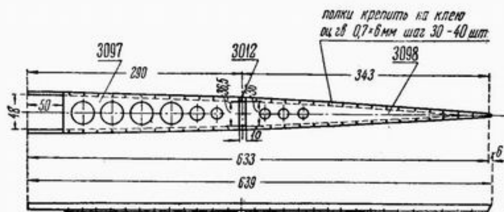
Рис. 131. Нервюра № 6 Габарит по теоретич. чертежу.
