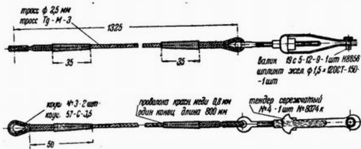
Рис. 221. Сгужной трос капота
