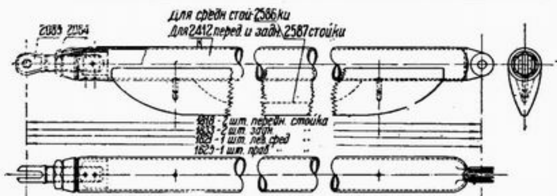
Рис. 104. Стойка коробки крыльев, 1-й вариант Окленть миткалевой лентой 50 мм на эмалите.
