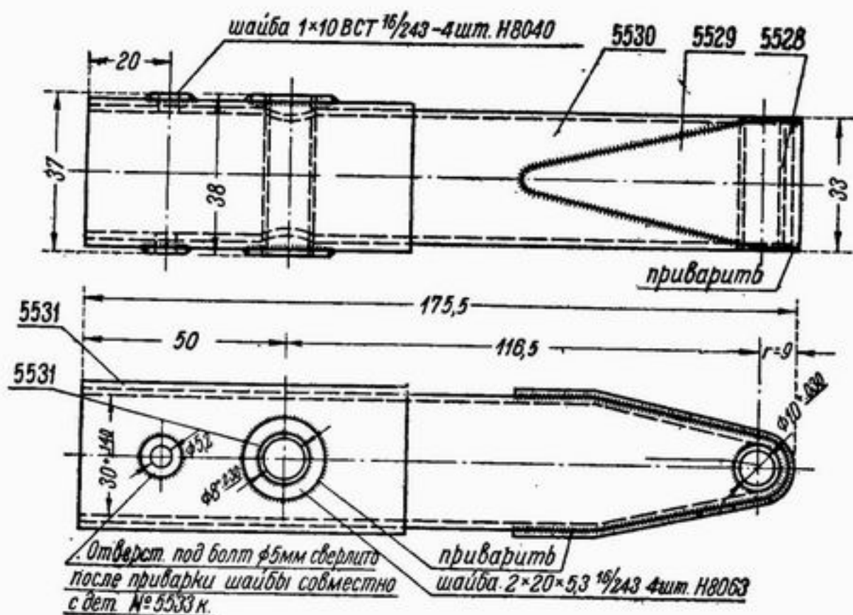
Рис. 140. Стакан ручки
