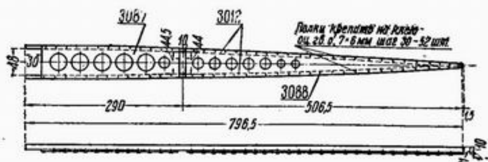
Рис. 129. Нервюра № 4 Габарит по чертежу.
