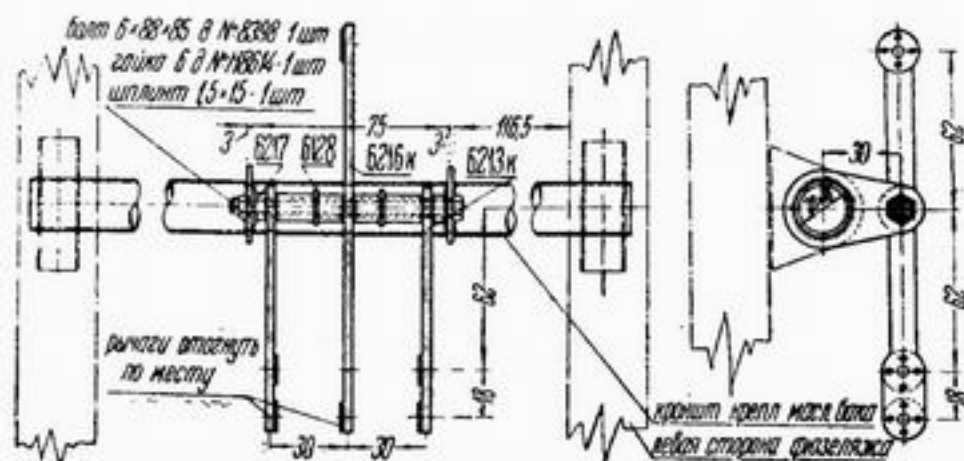
Рис. 212. Промежуточный мостик Рычаги устанавливать у левого борта.
