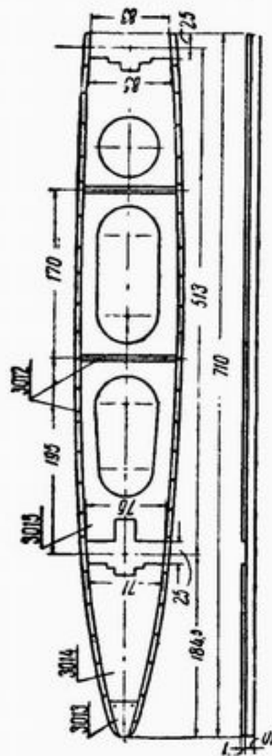
Рис. 112. Нормальная нервюра
