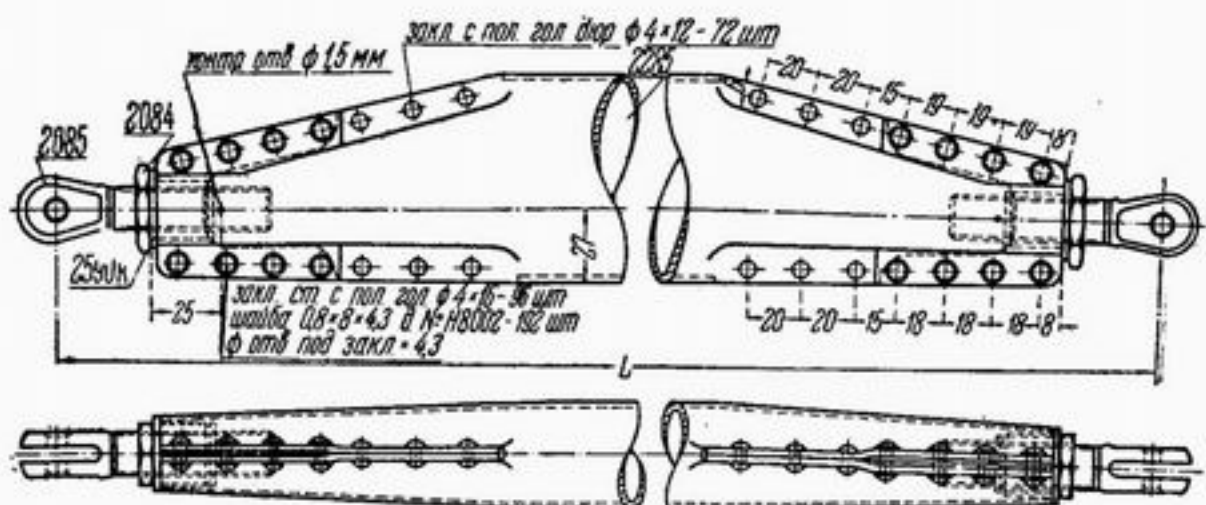
Рис. 107. Стойка коробки крыльев, 2-й вариант
