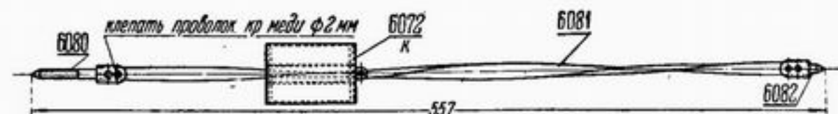
Рис. 199. Спираль бензиномера
