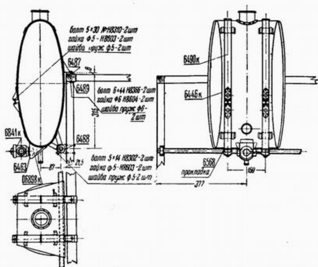
Рис. 201. Установка масляного бака
