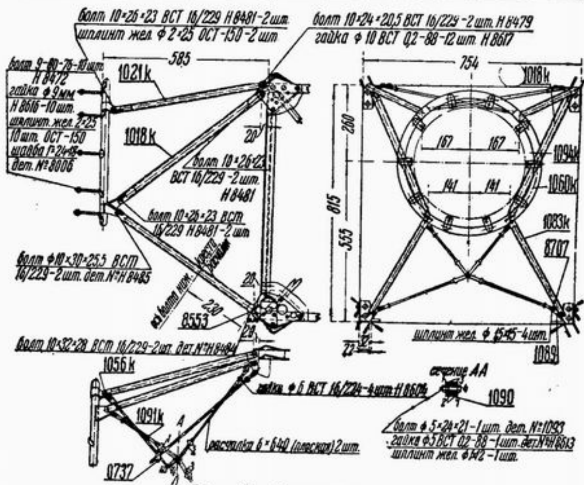
Рис. 65. Моторная рама
