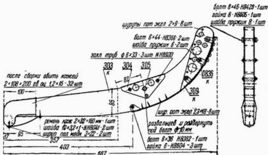
Рис. 172. Костыль
