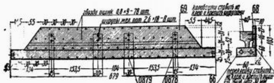
Рис. 20. Нижняя распорка № 1
