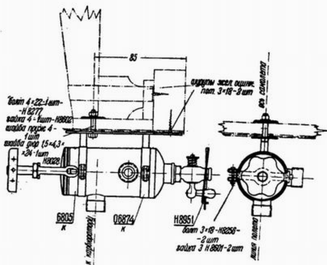
Рис. 195. Установка фильтра
