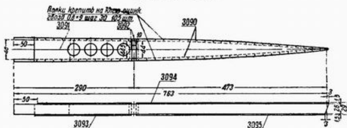
Рис. 129. Нервюра № 4 Габарит по чертежу.
