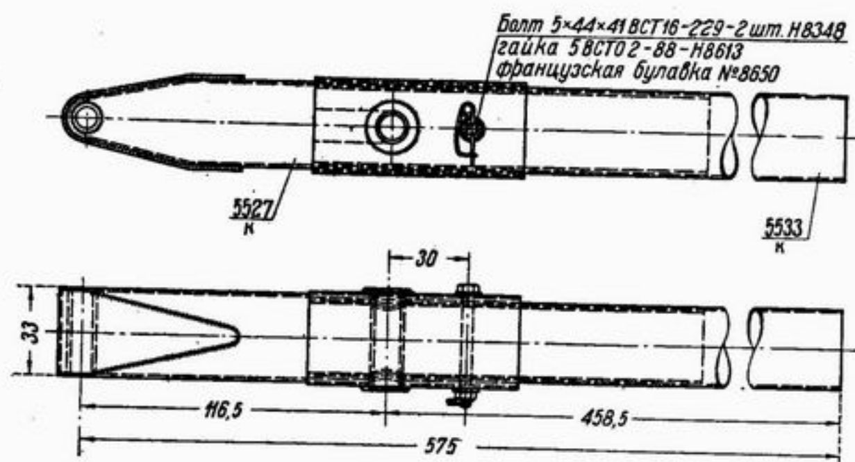
Рис. 139. Ручка управления
