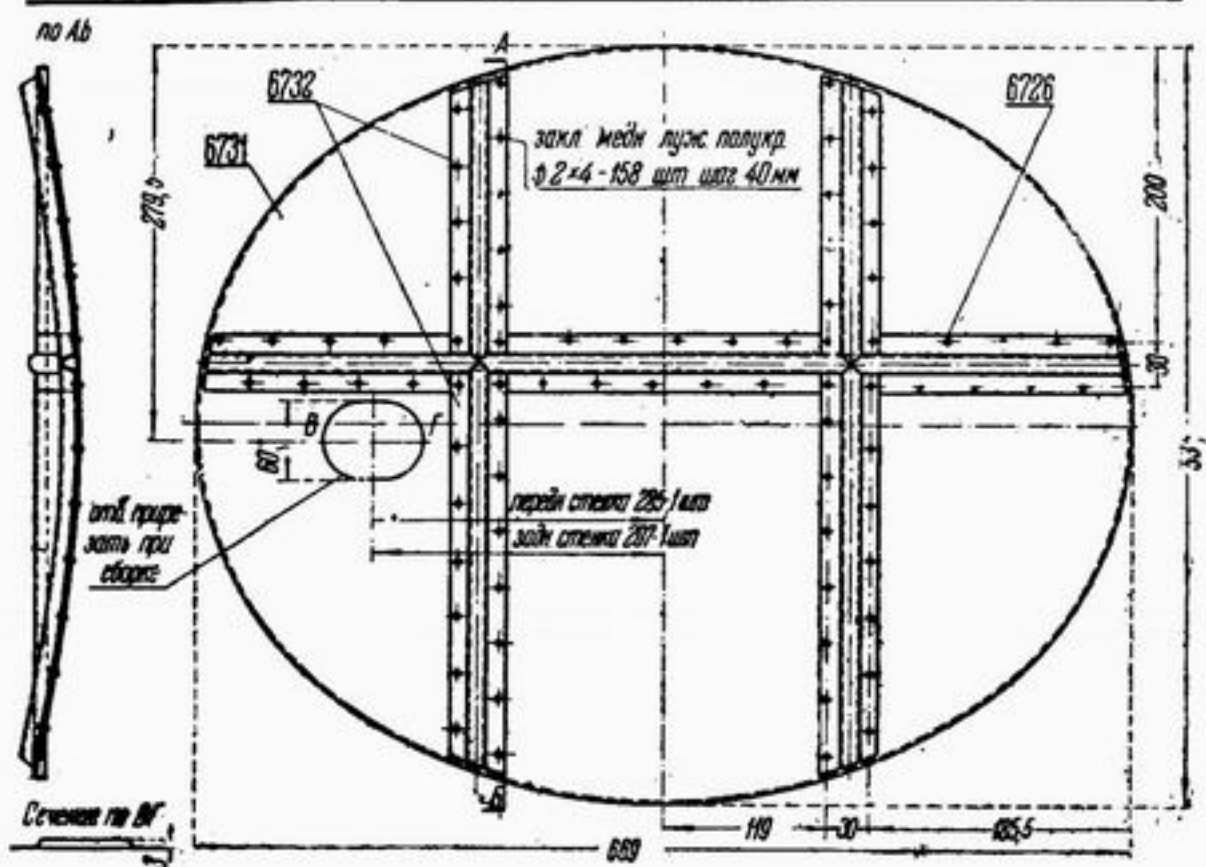
Рис. 187. Боковина бензинового бака
