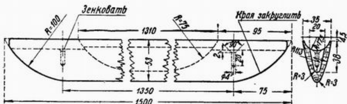
Рис. 106. Обтекатель стойки
