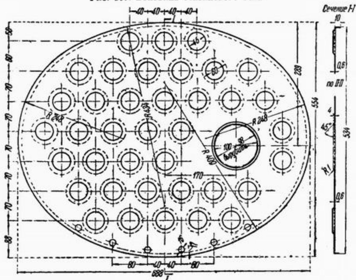
Рис. 188. Переборка бензинового бака
