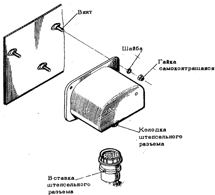
УСТАНОВКА БЛОКА БД-1
