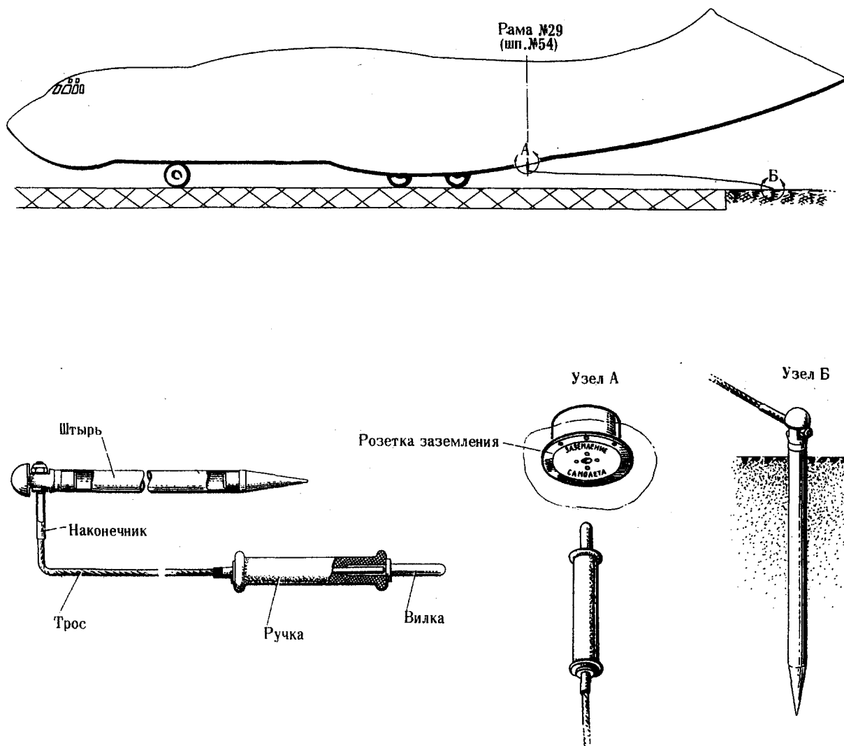
УСТРОЙСТВО ЗАЗЕМЛЕНИЯ САМОЛЕТА фиг. 5
