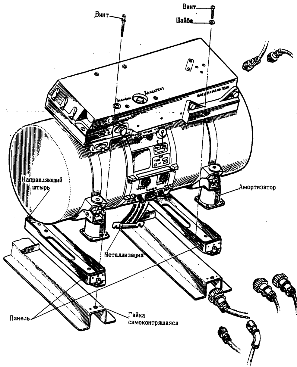
УСТАНОВКА ПРИБОРА П4-П-200 Фиг. 203
