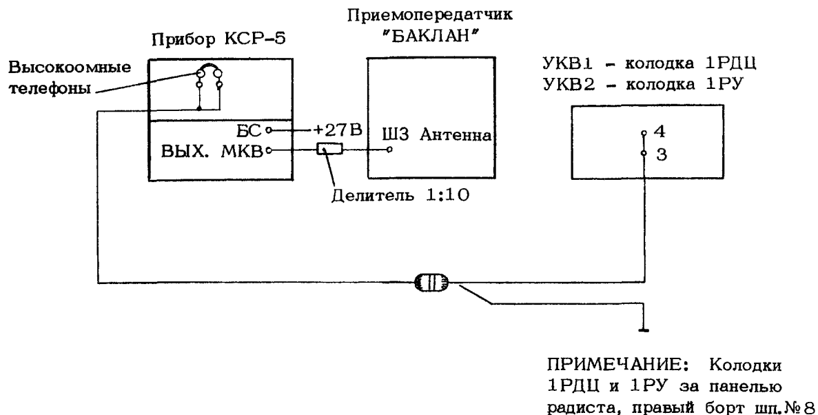
СХЕМА СОЕДИНЕНИЙ ДЛЯ ЗАМЕРА ЧУВСТВИТЕЛЬНОСТИ ПРИЕМНИКА
