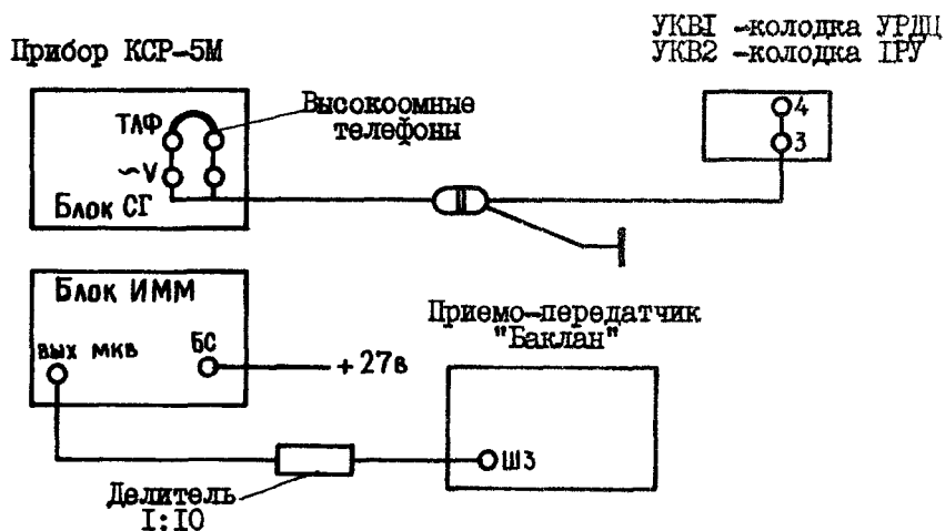
СХЕМА СОЕДИНЕНИЙ ДЛЯ ЗАМЕРА ЧУВСТВИТЕЛЬНОСТИ ПРИЕМНИКА фиг. 207
