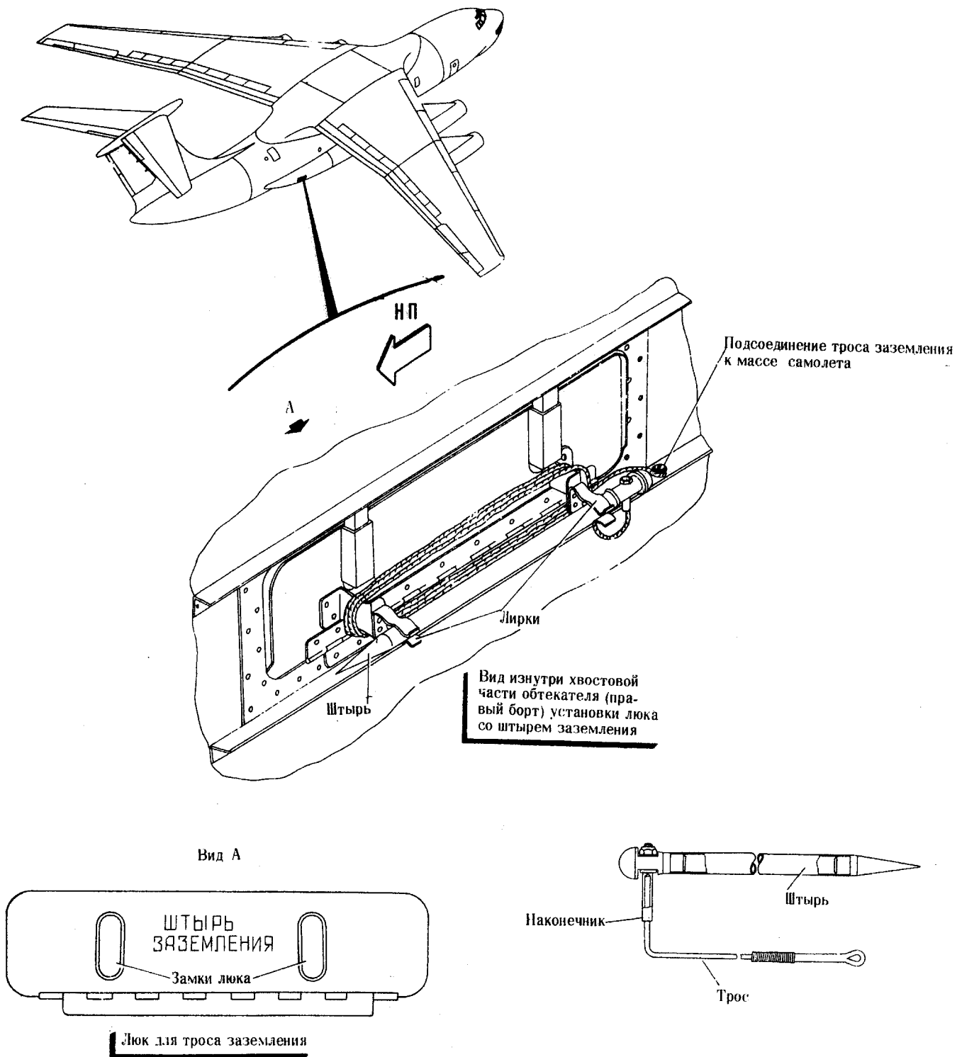
ШТЫРЬ ЗАЗЕМЛЕНИЯ САМОЛЕТА фиг. 4
