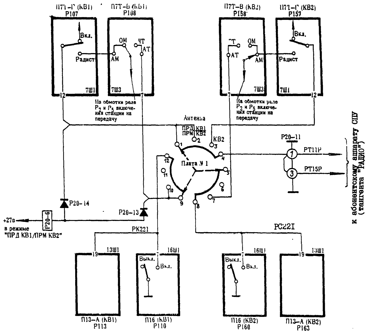
ПРИНЦИПИАЛЬНАЯ СХЕМА КОММУТАЦИИ ЦЕПЕЙ ЗАПУСКА ПЕРЕДАТЧИКОВ Фиг. 4
